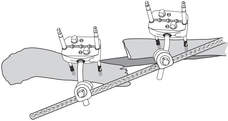
Рис. 22-13. Встановлення зовнішньої опори і двох міжпластинокових фіксаторів. Застосуйте поздовжнє витягування для репозиції перелому, встановіть зовнішню опору вздовж осі кістки і затягніть кріплення рами.
