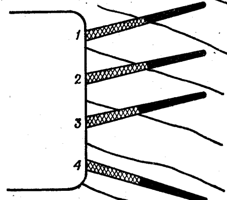
Рис. 334. Расположение шпуров в слоистых породах: а — нижний вруб; б — верхний вруб; 1 — врубовые шпуров; 2, 3 и 4 — отбойные шпуров
