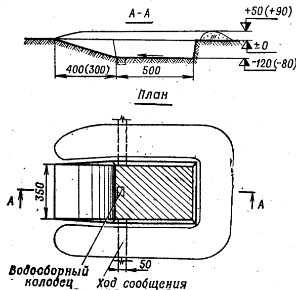
Рис. 54. Окоп для изде- лий 9П148, 9П136 (9П133)
