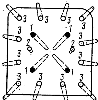
Рис. 332. Расположение шпуров при пирамидальном врубе: 1 — врубовые шпуров; 2 и 3 — отбойные шпуров
