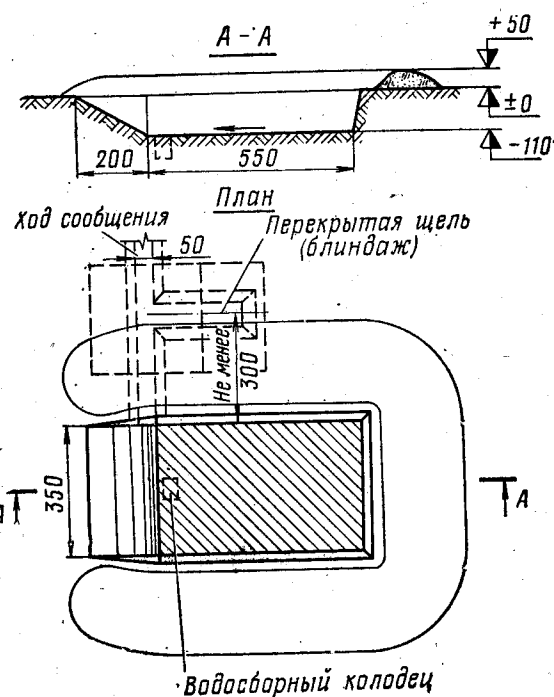
Рис. 77. Окоп для зенитных самоходных артиллерийских установок ЗСУ-23-4 и ЗСУ-57-2
