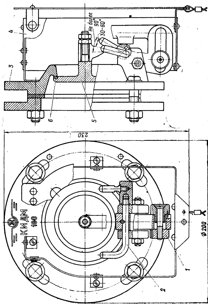
Рис. 278. Клапан избыточного давления КИДМ-100: 1 — противовес; 2 — рычаг стопора; 3 — корпус; 4 — кожух; 5 — тарелка; 6 — прокладка
