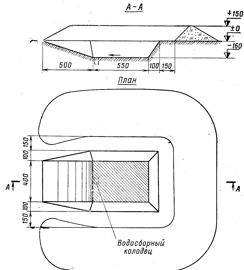
Рис. 73. Окоп для изделия 2П25
