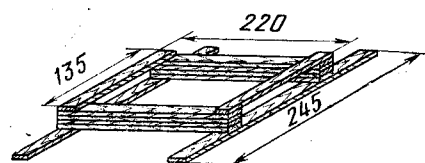
Рис. 375. Укладка комплекта сооружения СПС-2М на автомобиль КраЗ-255Б (КраЗ-260) при транспортировании: 1 — элемент ПС1ад; 2 — элементы ПС3; 3 — элементы КЗ; 4 — колья; 5 — металлическая защитно-герметическая дверь ДЗГМ-50×100 — 2 шт.; 6 — элементы ПС2; 7 — щиты пола; 8 — подставка для элемента ПС1ад
