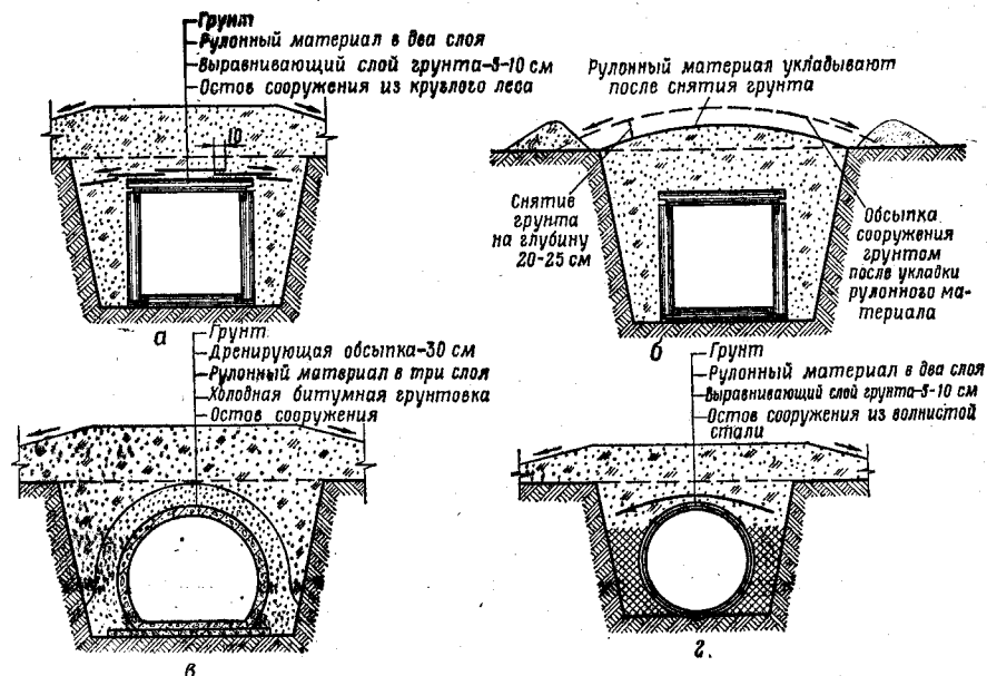
Рис. 239. Гидроизоляция и герметизация остовов сооружений закрытого типа рулонным материалом:
