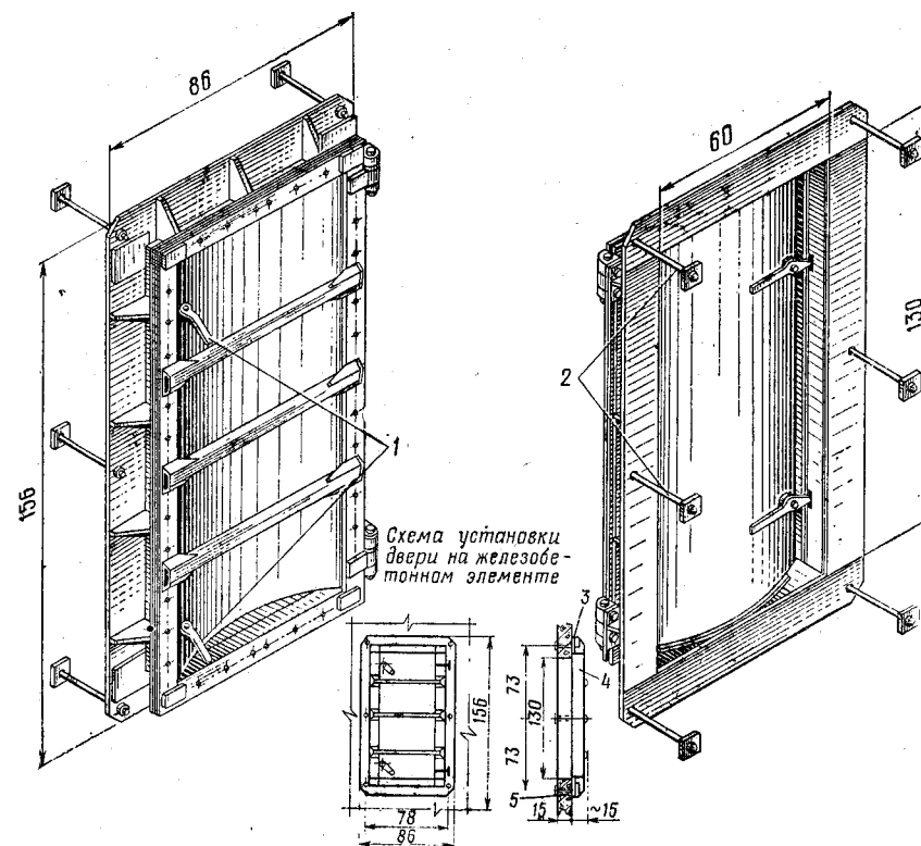
Рис. 251. Дверь защитная металлическая ДЗМ; масса 158 кг:
