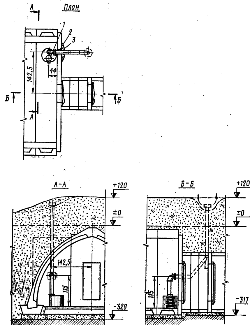
Рис. 286. Установка ОП в сооружении УСВ:
