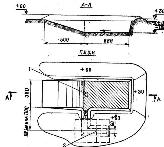
Рис. 26. Окоп для бронетранспортера:
