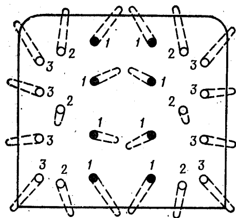
Рис. 333. Расположение шпуров при клиновом врубе: а — вертикальный вруб; б — горизонтальный вруб; 1 — врубовые шпуров; 2 и 3 — отбойные шпуров
