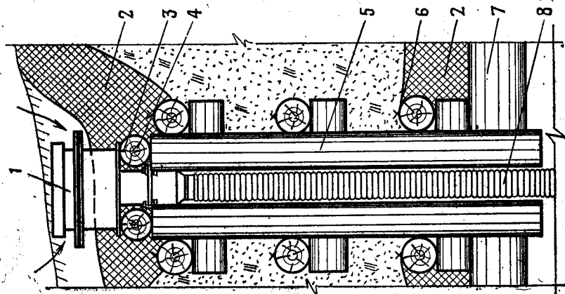
Рис. 268. Короб из круглого леса для пропуска воздухозаборного шланга ФВА-50/25:
