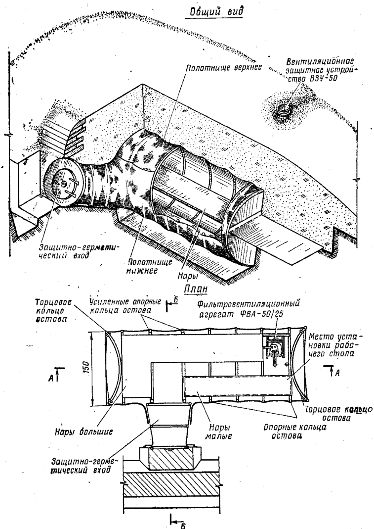
Рис. 128. Легкое каркасное сооружение ЛКС-2
