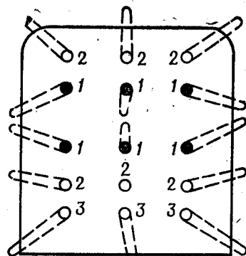
Рис. 333. Расположение шпуров при клиновом врубе: а — вертикальный вруб; б — горизонтальный вруб; 1 — врубовые шпуров; 2 и 3 — отбойные шпуров
