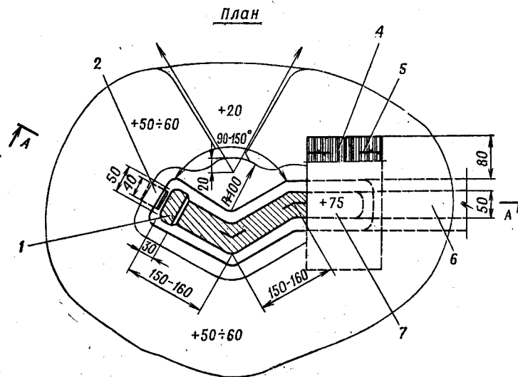
Рис. 383. Окоп для стрельбы из пулемета стоя с нишей на одного человека:
