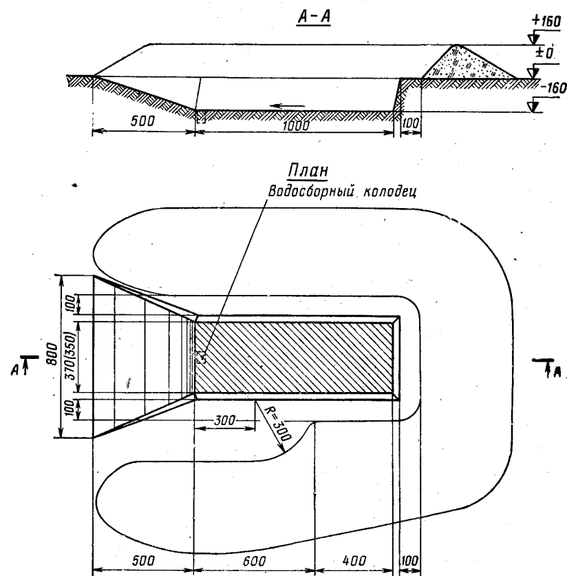
Рис. 69. Окоп для изделия 9П140
