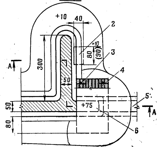
План
