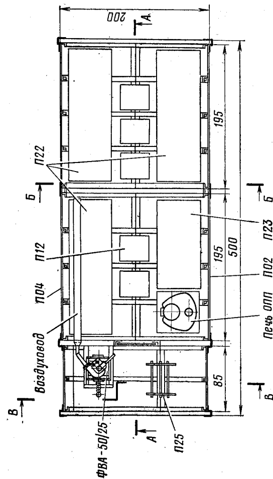
Рис. 132. Быстроизвлекаемое метал- лическое сооружение «Пакет» (об- щий вид, план)
