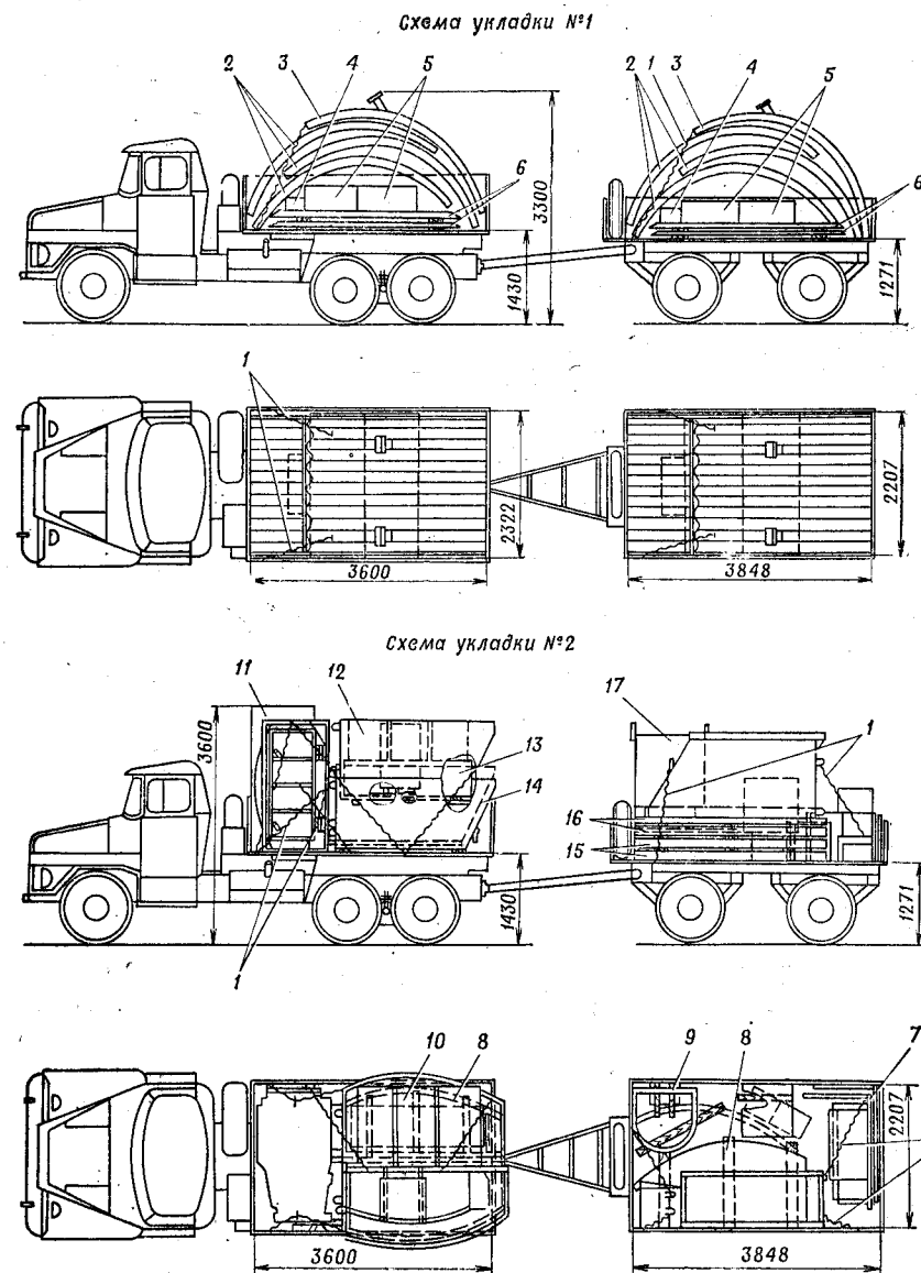
Рис. 379. Укладка комплекта сооружения «Бункер» на два автомобиля ЗИЛ-131 с прицепами ИАПЗ-754В при транспортировании:
