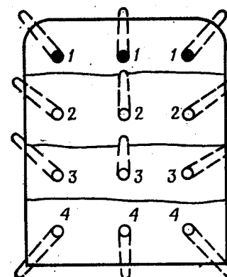
Рис. 334. Расположение шпуров в слоистых породах: а — нижний вруб; б — верхний вруб; 1 — врубовые шпуров; 2, 3 и 4 — отбойные шпуров
