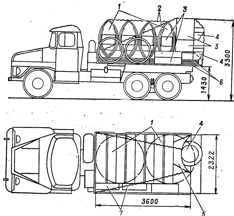
Рис. 377. Укладка двух комплектов сооружения «Пакет» на автомобиль ЗИЛ-131 при транспортировании:
