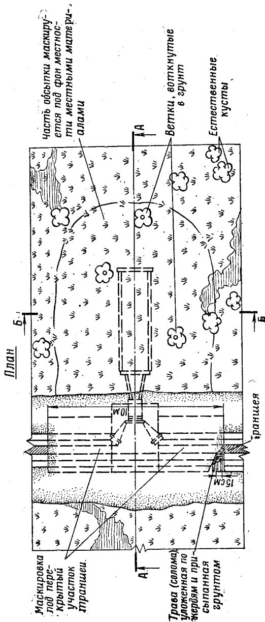
Рис. 125. Маскировка убежища под фон окружающей местности На маскировку убежища требуется 12 чел.-час., жердей d=7 см — 150 м
