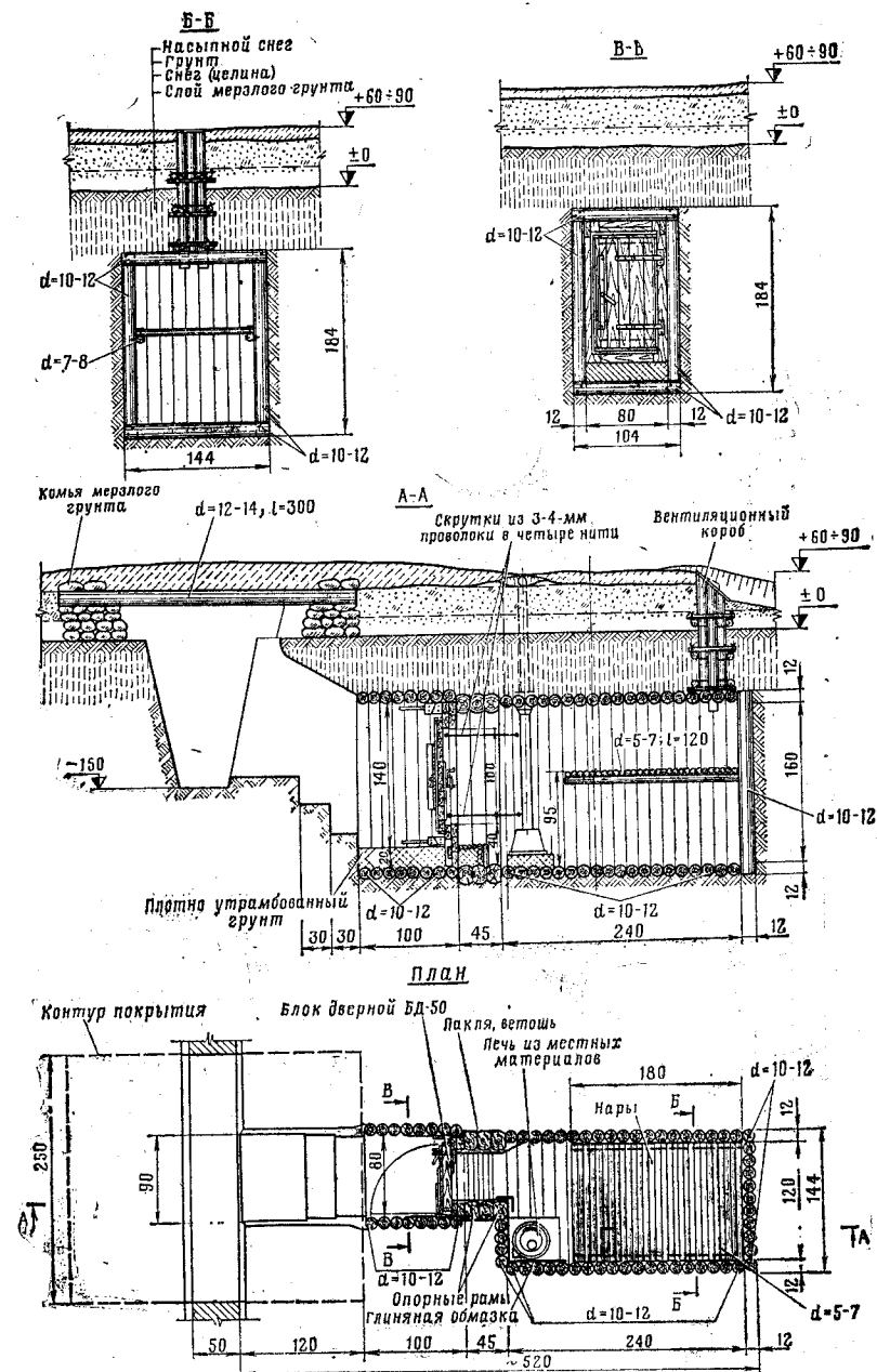
Рис. 199. Блиндаж из бревенчатых рам, возводимый под слоем мерзлого грунта Объем вынутого грунта 12 м³. На устройство блиндажа требуется 136 чел.-час., лесоматериала — 3,6 м³
