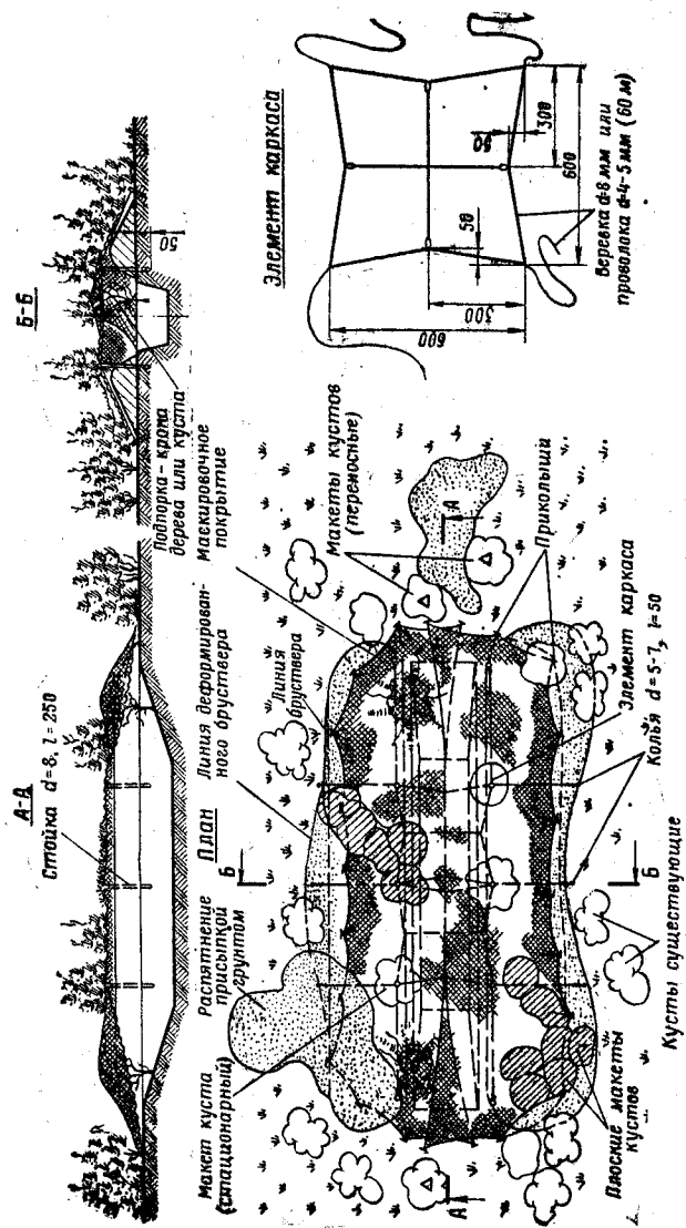
Рис. 180. Маскировка укрытия для крупногабаритной техники
