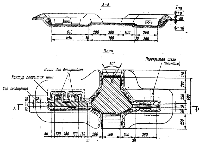
Рис. 222. Окоп с ограниченным сектором обстрела и одеждой крутостей из БЗМ-57 для 100-мм пушки
