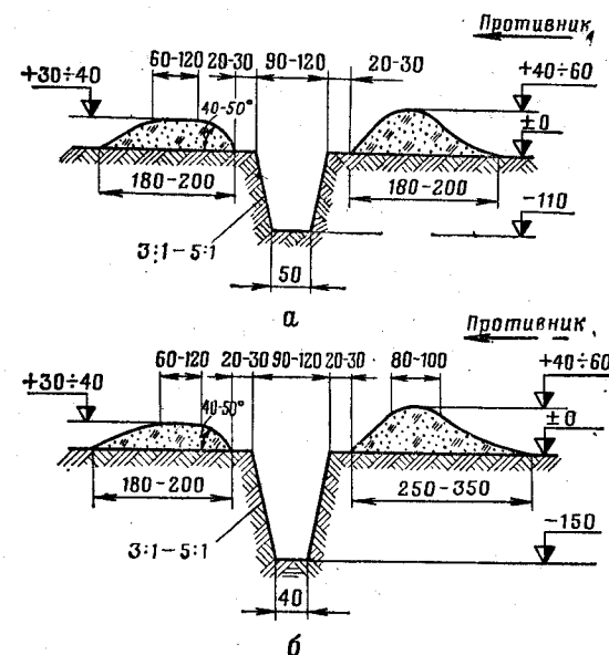
Рис. 17. Профили траншей и ходов сообщения, отрываемых вручную: а — основной. Объем вынутого грунта с 1 м траншеи 0,8 м 3 . На устройство 1 м траншеи требуется 0,8 чел.-час.; б — полный. Объем вынутого грунта с 1 м траншеи 1,1 м 3 . На устройство 1 м траншеи требуется 1,2 чел.-час.
