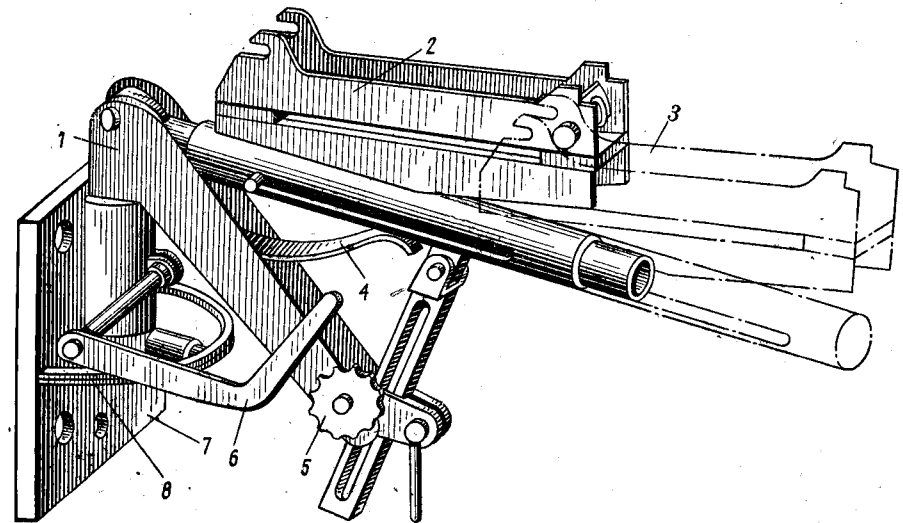
Рис. 255. Пулеметный станок СПН; масса 12 кг: 1 — вертлюг; 2 — постель станка; 3 — крайнее заднее положение постели станка; 4 — уравнивающий механизм; 5 — механизм вертикальной наводки; 6 — рукоятка механизма горизонтальной наводки; 7 — привалочный фланец; 8 — сектор горизонтальной наводки
