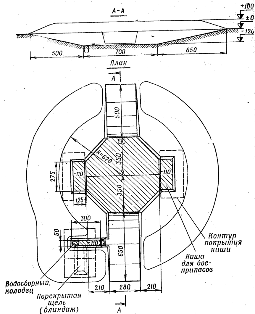
Рис. 79. Окоп для 100-мм зенитной пушки КС-19 Объем вынутого грунта 85 м³. На устройство окопа (без щели) требуется 0,9 маш.-час. экскаватора ЭОВ-4421 и 25 чел.-час.; вручную — 105 чел.-час.
