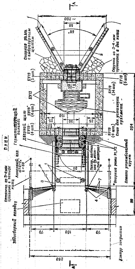
Рис. 184. Сборное пулеметное сооружение из железобетонных перемишек Объем вынутого грунта 18 м 3 . На устройство сооружения требуется 0,2 (0,8) маш.-час. экскаватора ЭОВ-4421 (Э-305Б) и 110 чел.-час., железобетона — 3,4 м 3 , лесоматериала — 2,7 м 3 , проволоки — 10 кг
