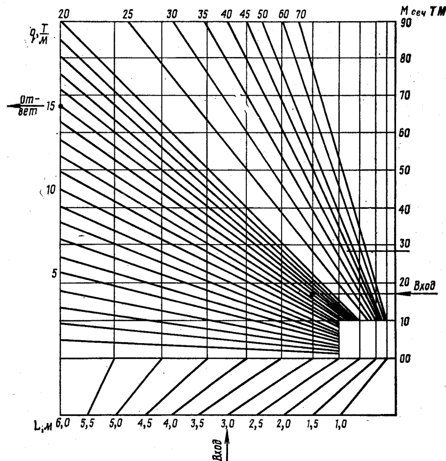
Рис. 4. Номограмма для определения q_{экв}
