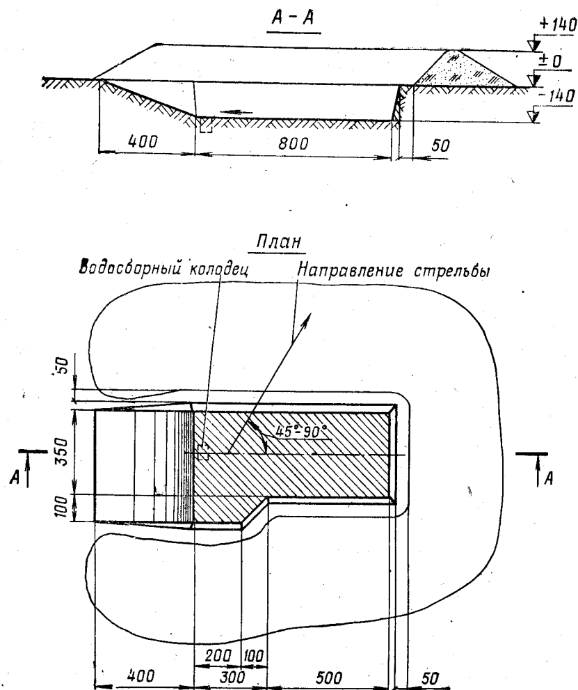
Рис. 70. Окоп для изделий 9П138 и БМ-21 Объем вынутого грунта 60 м³. На устройство окопа требуется 0,8 маш.-час. ПЗМ-2 и 16 чел.-час.
