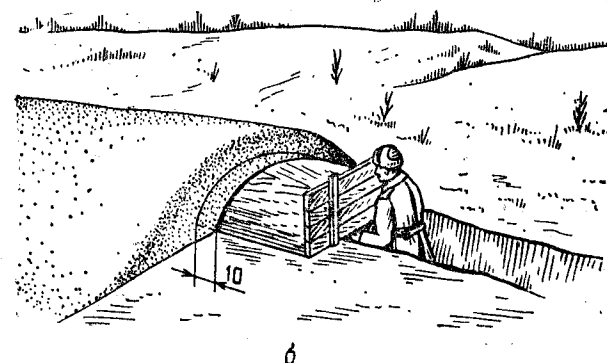
Рис. 193. Устройство свода из снега с помощью передвижной опалубки:
