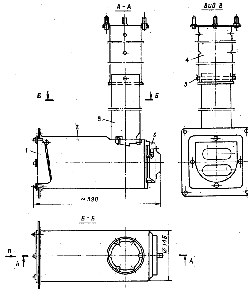
Рис. 277. Устройство для продувки тамбуров ППУ:
