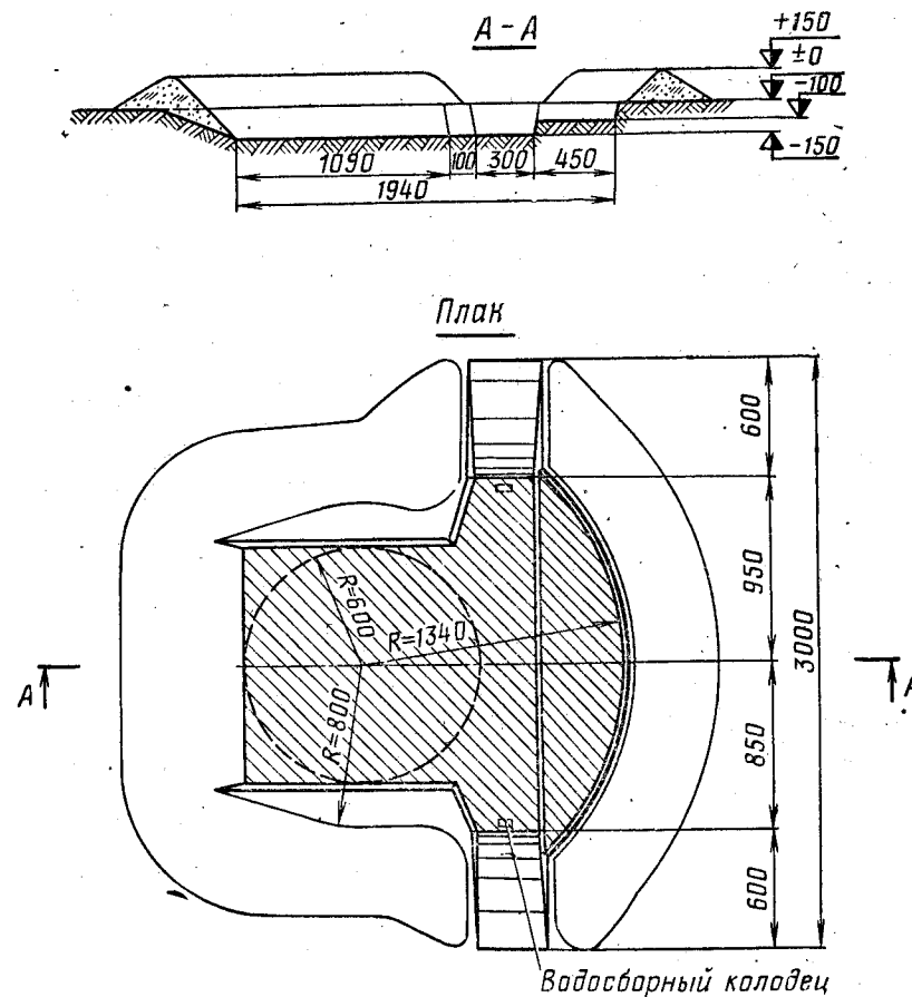
Рис. 75. Окоп для пусковой установки комплекса С-75 Объем вынутаго грунта 390 м³. На устройство окопа требуется 10 маш.-час. на-весного бульдозерного оборудования и 10 чел.-час.
