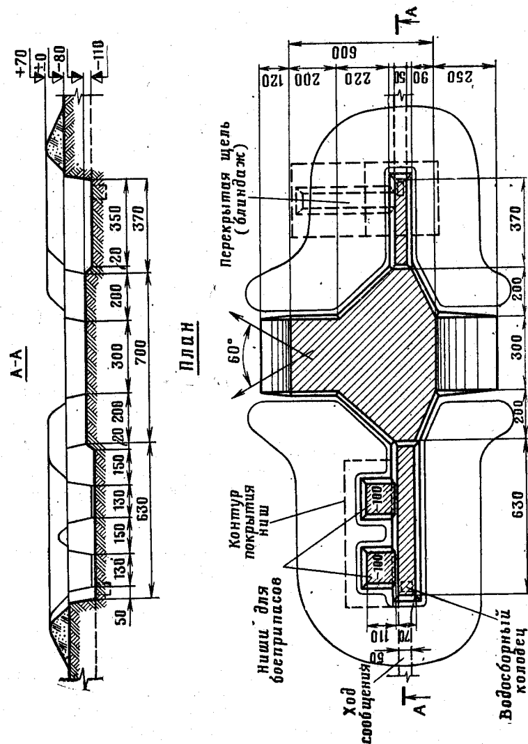
Рис. 56. Окоп с ограниченным сектором обстрела для 100-мм пушек МТ-12 и Т-12. Объем вынутого грунта 40 м³. На устройство окопа (без щели) требуется 0,4 маш.-час. экскаватора ЭОВ-4421 и 18 чел.-час.; вручную — 53 чел.-час.
