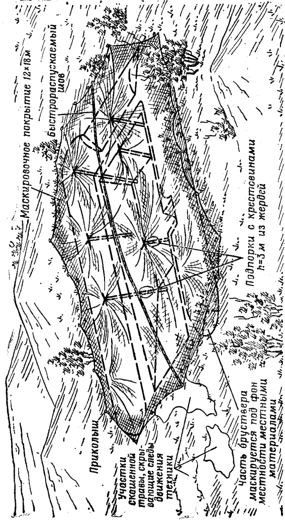
Рис. 46. Маскировка окопов для боевой техники под фон местности На маскировку требуется 2 чел.-час., маскировочных покрытий 12 \times 18 м — 1 шт., жердей d=5-7 см — 18 м, приколышей — 24 шт., гвоздей — 20 шт.
