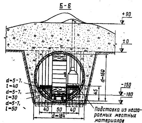
Рис. 186. Блиндаж из железобетонной трубы и перемычек (разрез)
