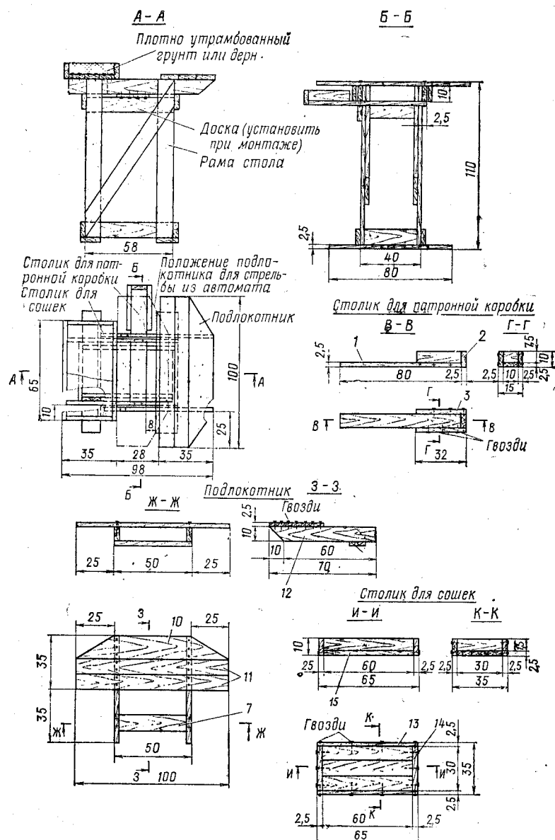
Рис. 363. Стол для установки пулемета в сборном пулеметном сооружении из железобетонных перемычек
