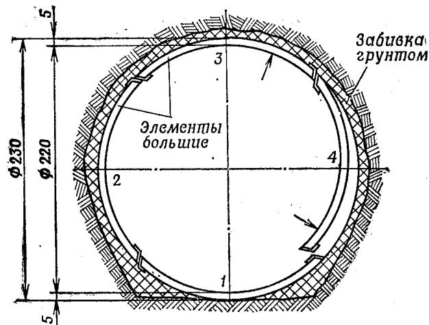
Рис. 331. Последовательность (1—4) установки элементов КВС-А-1 в подземной выработке
