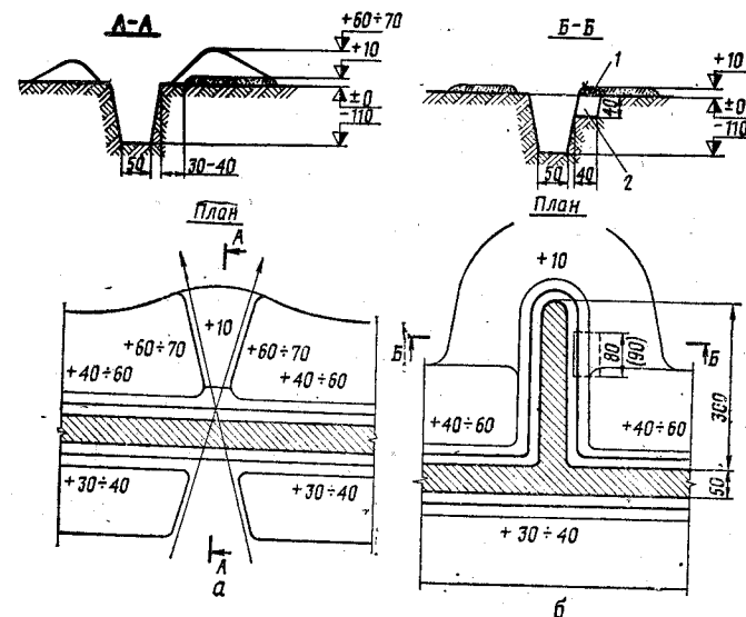
Рис. 22. Оборудование траншеи для стрельбы из ручного противотанкового гранатомета (реактивного пехотного огнемета):
