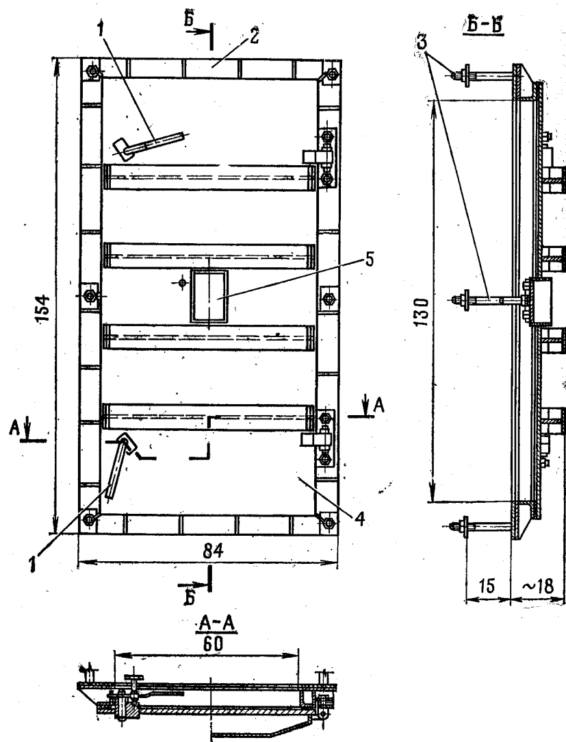
Рис. 250. Дверь защитно-герметическая металлическая ДЗГМ-60×130-3; масса 214 кг:
