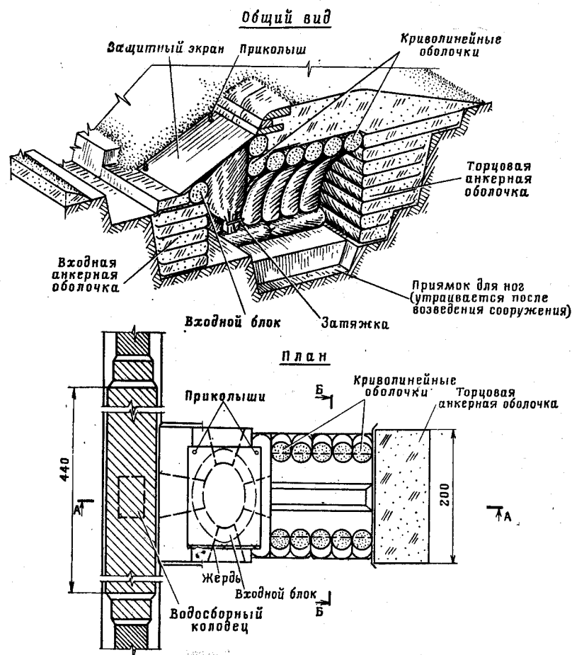
Рис. 232. Сооружение из криволинейных оболочек «Оболочка-1» Объем вынутого грунта 15 м³. На устройство сооружения требуется 24 чел.-час., «Оболочка-1» — 1 компл.; время на извлечение — 12 чел.-час.
