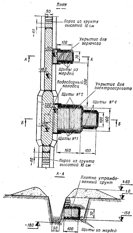
Рис. 167. Укрытие для электроагрегата АБ-2 Объем вынутого грунта 16 м 3 . На устройство укрытия
