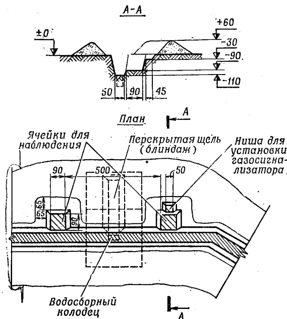
Рис. 104. Открытое сооружение для инженерного (химического) наблюдательного поста. Объем вынутого грунта 7,5 м³. На устройство сооружения (без щели) требуется 9 чел.-час.
