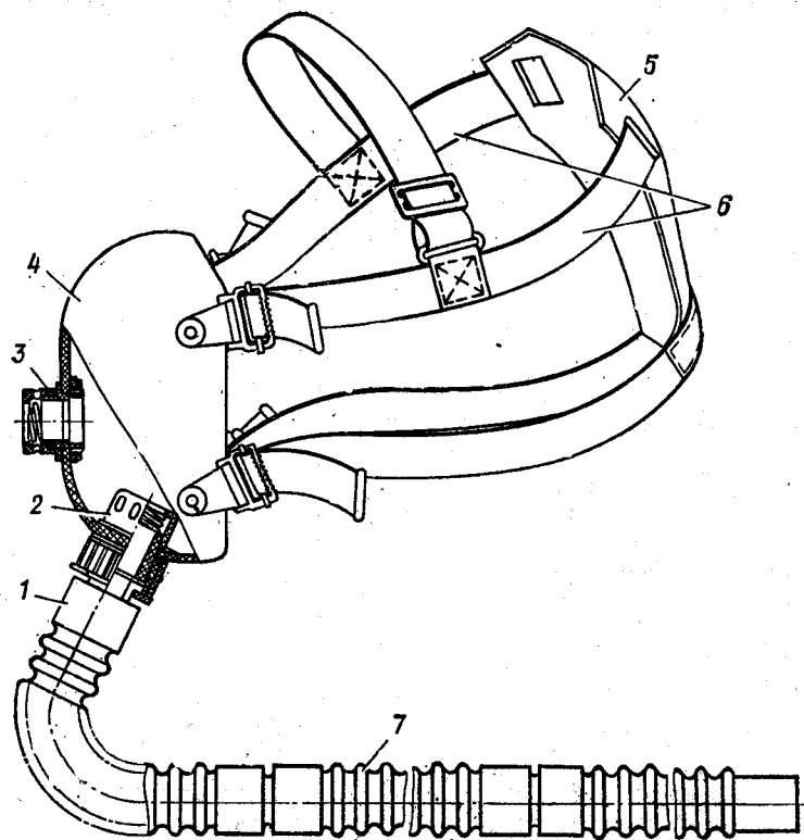
Рис. 263. Полумаска ПФС:
