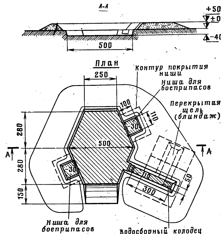
Рис. 78. Окоп для 57-мм зенитной пушки С-60
