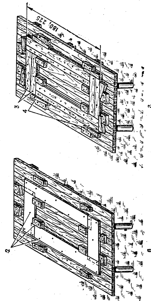
Рис. 372. Последовательность сборки герметических перегородок 100×180 см, 120×225 см и 150×225 см:
