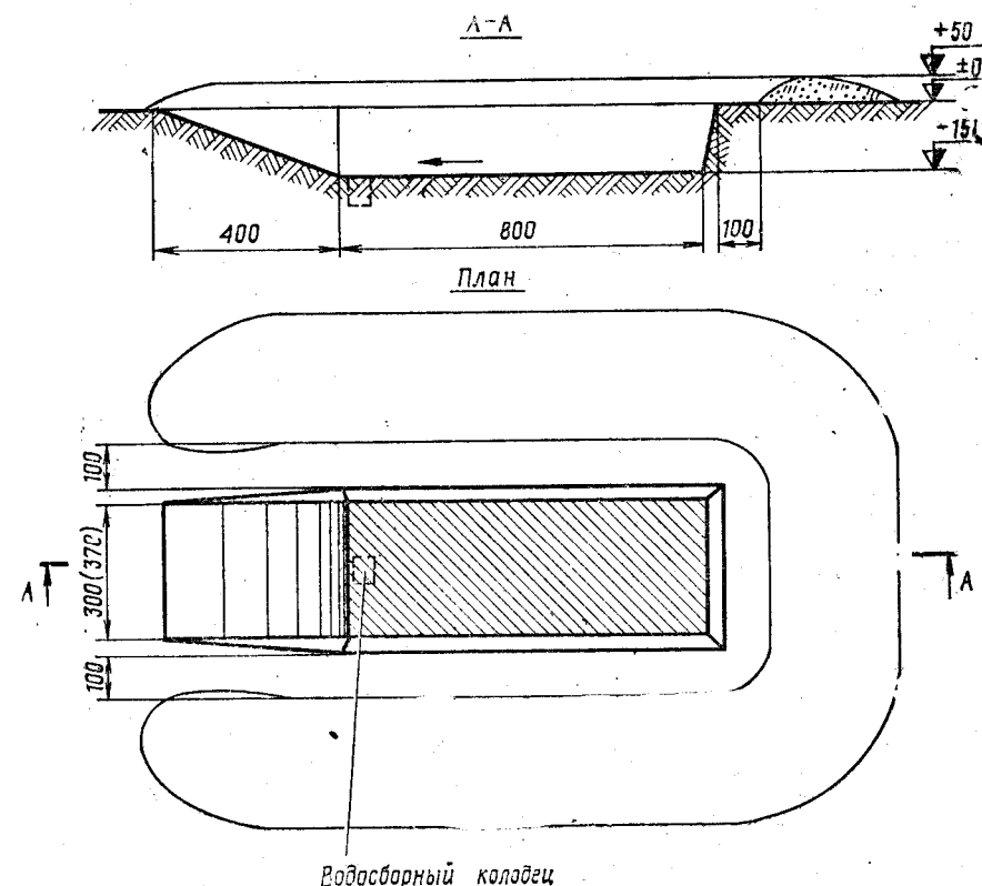
Рис. 71. Окоп для изделия 9А33Б Объем вынутого грунта 50 (60) м³. На устройство окопа требуется 0,5 (0,2) маш.-час. экскаватора ЭОВ-4421 (МДК-3) и 12(5) чел.-час.
