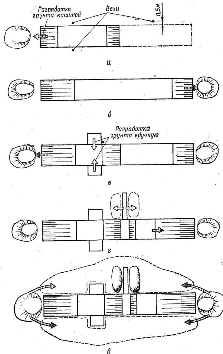
Рис. 309. Последовательность отрывки окопа для 240-мм миномета с помощью навесного бульдозерного оборудования:
