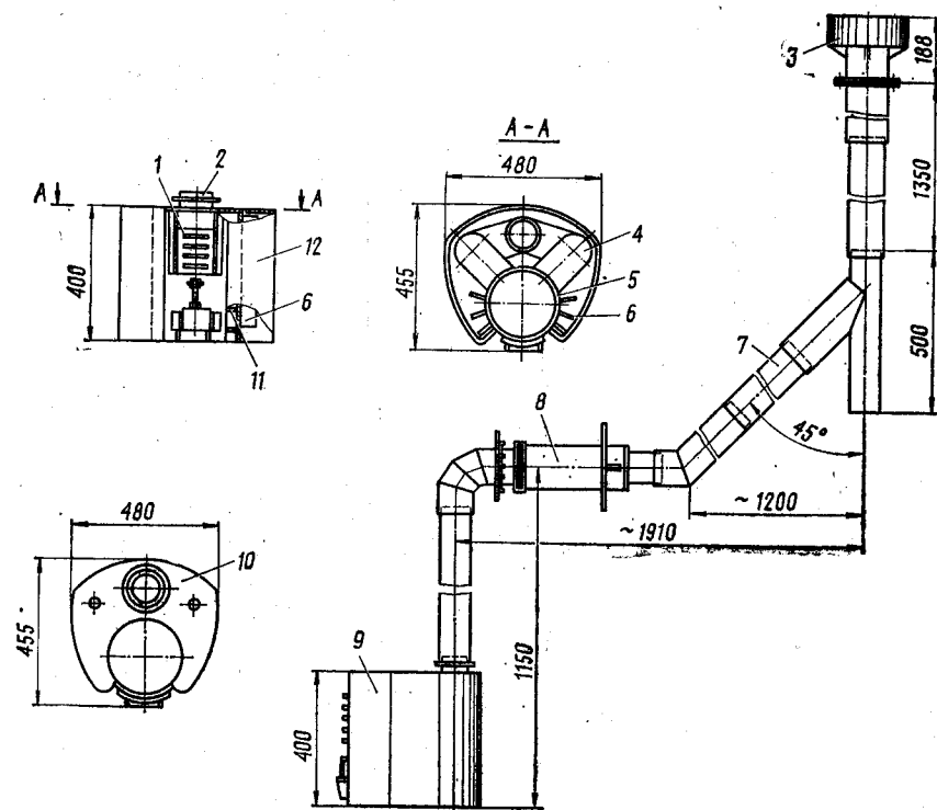
Рис. 281. Обогревательная полевая печь ОПП:
