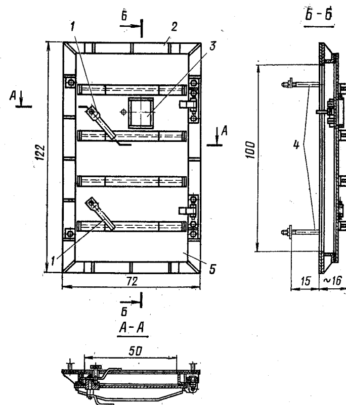
Рис. 249. Дверь защитно-герметическая металлическая ДЗГМ-50×100-2; масса 151 кг: 1 — задрайка; 2 — опорная рама; 3 — заслонка бойницы; 4 — крепежные болты; 5 — полотно двери
