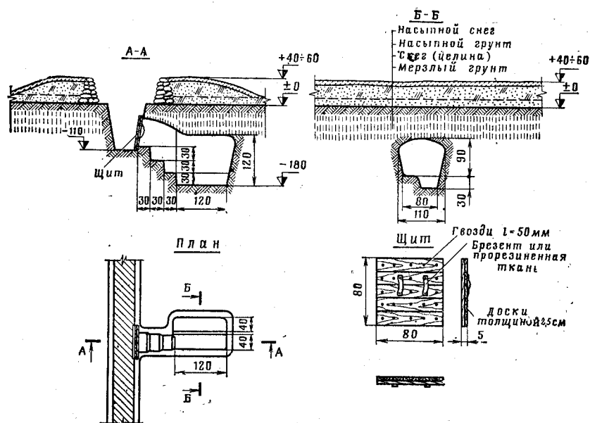
Рис. 196. Ниша для двух человек, устраиваемая под слоем мерзлого грунта Объем вынутого грунта 1,5 м 3 . На устройство ниши требуется 13 чел.-час.
