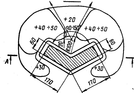
Рис. 7. Окоп для стрельбы из пулемета с колена
