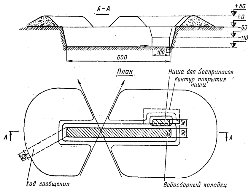
Рис. 55. Окоп для станкового противотанкового гранатомета СПГ-9М. Объем вынутого грунта 5 м³. На устройство окопа пехотной лопатой требуется 10 чел.-час., саперной лопатой — 7 чел.-час.
