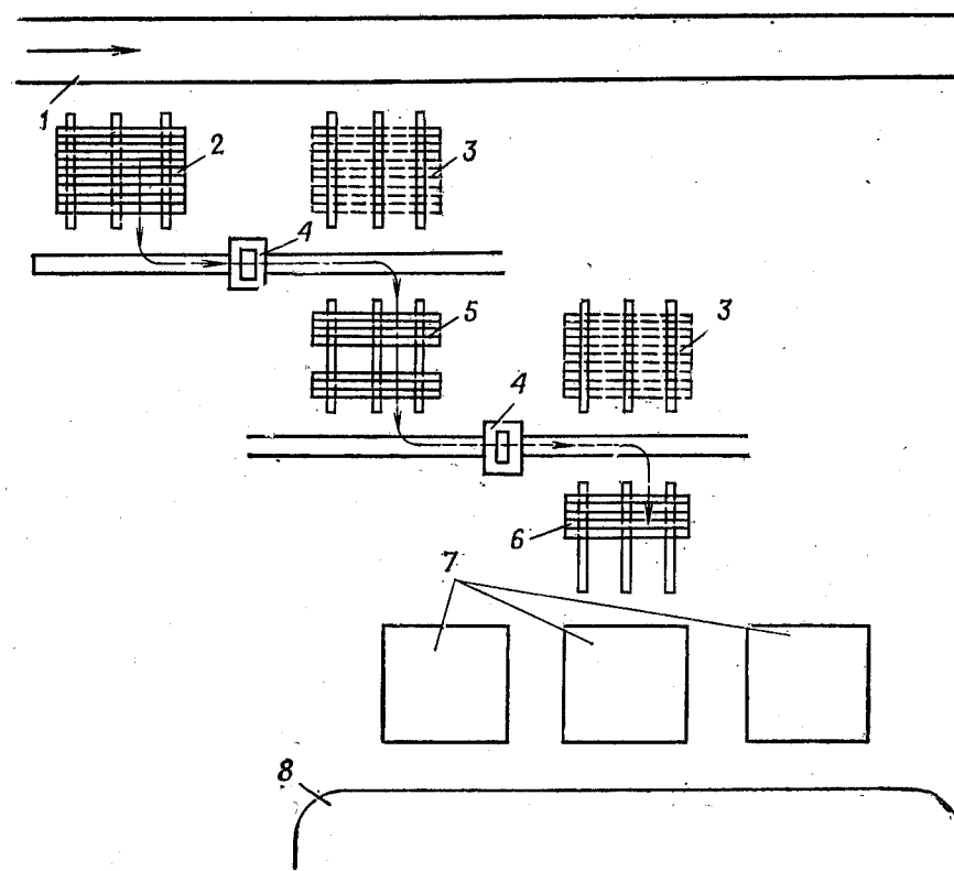
Рис. 337. Лесозавод с последовательным расположением лесопильных рам: 1 — путь подвоза бревен; 2 — эстакада для подачи бревен; 3 — запасная эстакада для подачи бревен; 4 — лесопильная рама ЛРВ-1; 5 — эстакада для приема двухкантных брусков; 6 — эстакада для приема пиломатериалов; 7 — склады пиломатериалов; 8 — механизированная площадка заготовки деталей и конструкций из пиломатериалов
