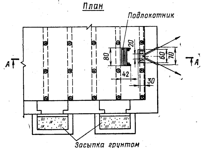
Рис. 183. Приспособление подвала здания для стрельбы из пулемета
