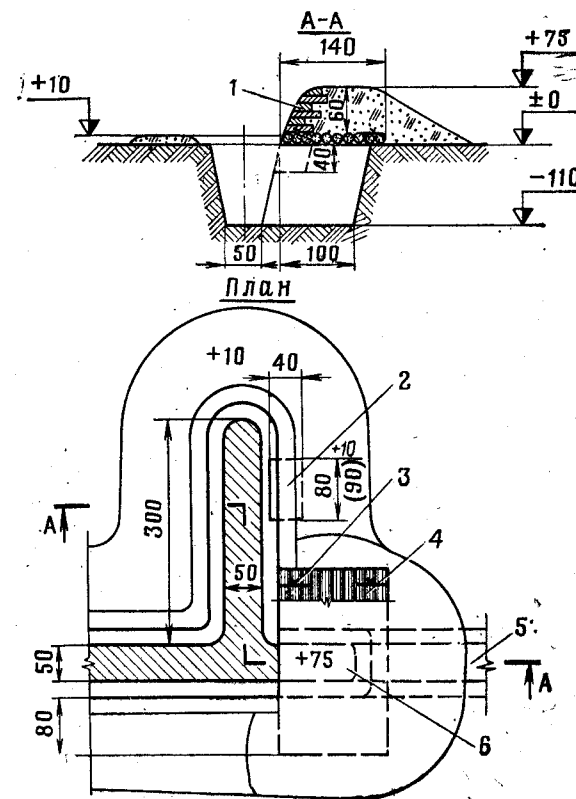
Рис. 384. Окоп для стрельбы из ручного противотанкового гранатомета (реактивного пехотного гранатомета) с нишей на одного человека:
