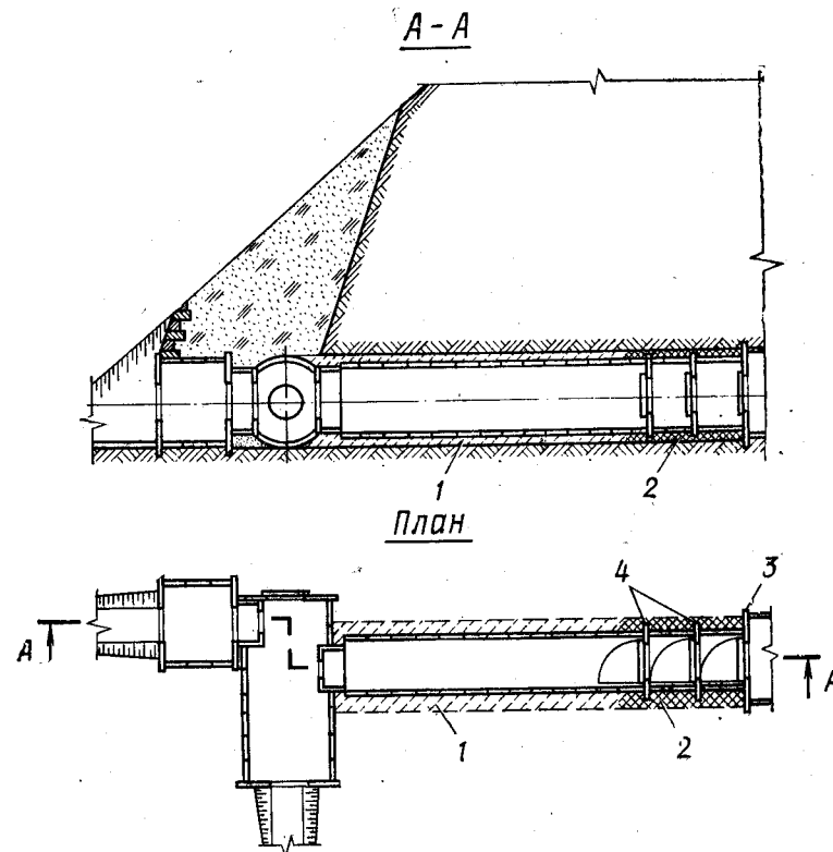
Рис. 302. Герметизация входов в подземные сооружения:
