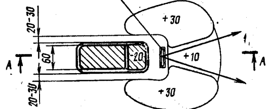
Рис. 6. Окоп для стрельбы из пулемета лежа
