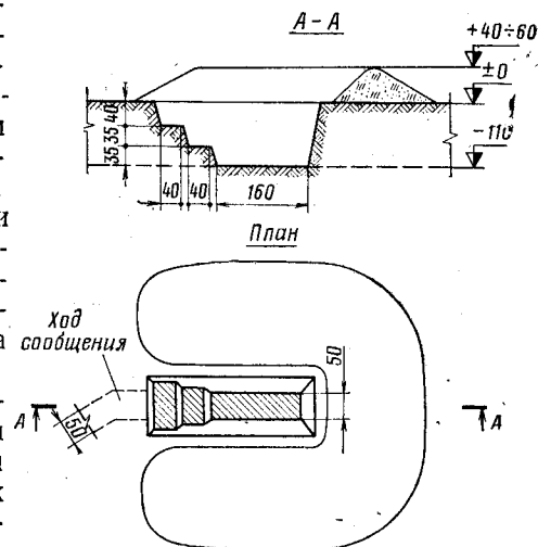
Рис. 95. Открытое сооружение для командира огневого взвода
