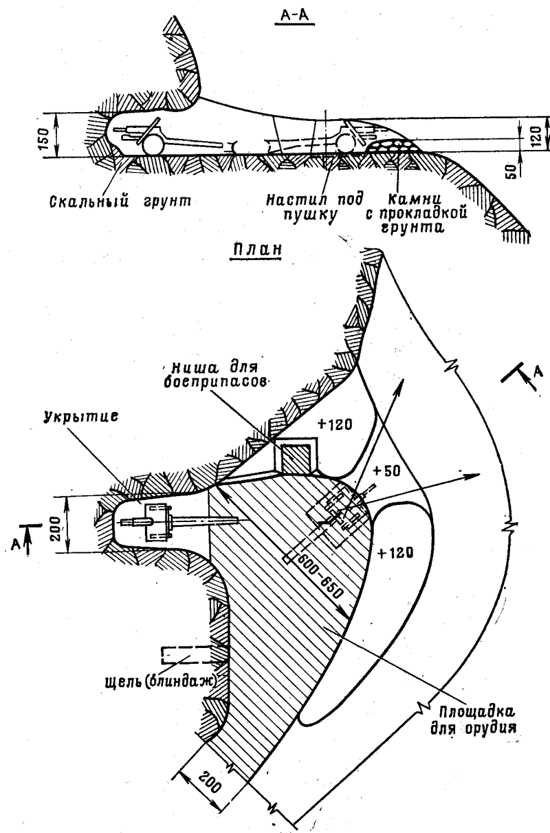
Рис. 215. Окоп с укрытием для 76-мм пушки, устраиваемый на переднем скате в горах На устройство окопа требуется 40 чел.-час., камня — 10 м³
