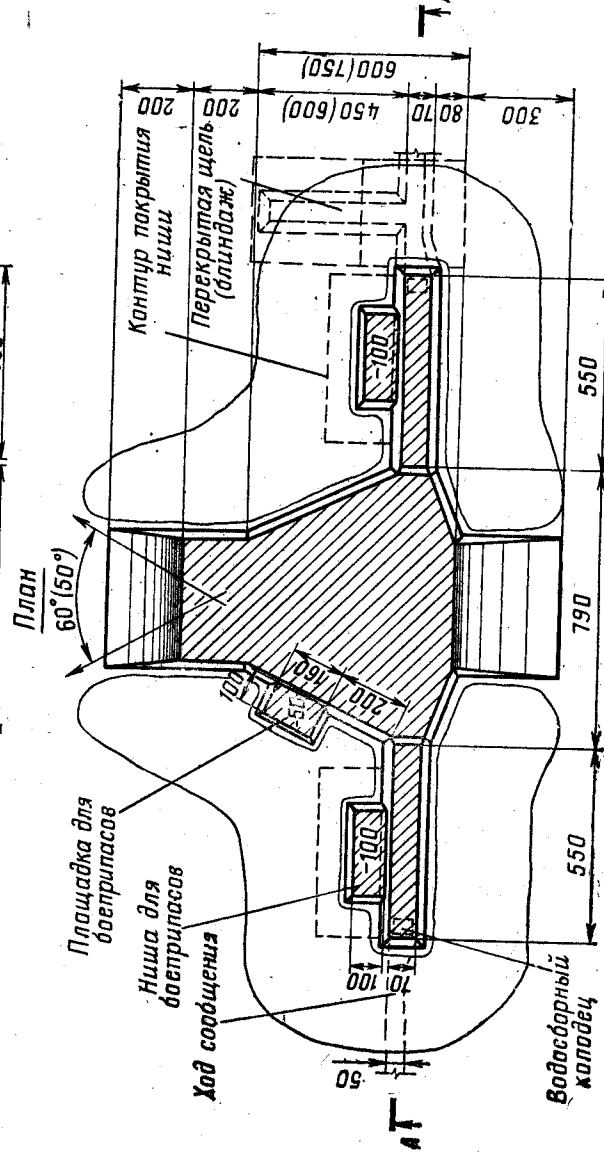
Рис. 60. Окоп для 152-мм пушки-гаубицы Д-20 и изделия 2А36 Объем вынутаго грунта 65(75) м 3 . На устройство окопа (без щели) требуется 12(11,4) маш.-час. АТС и 35(38) чел.-час.; вручную — 82(95) чел.-час. Примечания: 1. Для пушки-гаубицы Д-20 правая ниша не устраивается. 2. Цифры в скобках относятся к окопу для изделия 2А36
