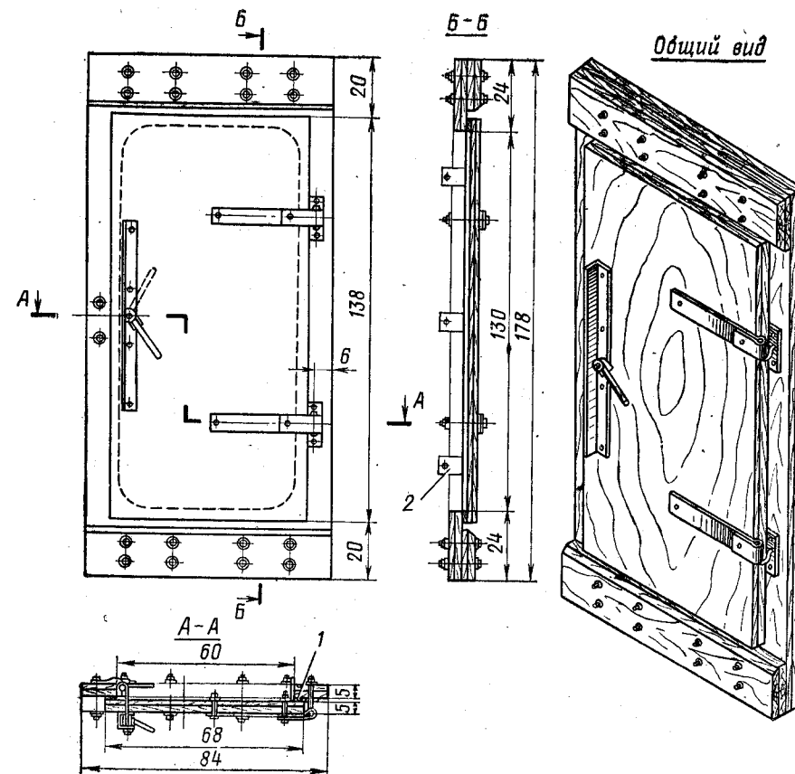
Рис. 247. Блок дверной фанерный БДФ; масса 90 кг: 1 — герметизирующая прокладка; 2 — металлическая накладка
