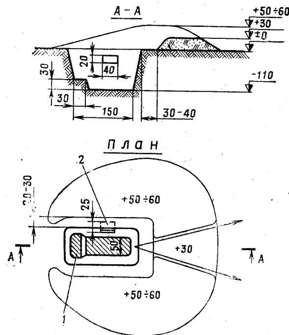
Рис. 4. Окоп для стрельбы из автомата стоя:
