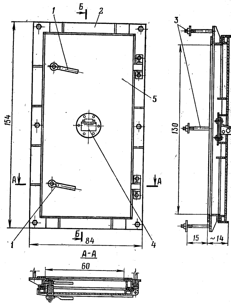
Рис. 252. Дверь герметическая ДГМ; масса 100 кг: 1 — задрайка; 2 — опорная рама; 3 — крепежные болты; 4 — клапан перетекания воздуха; 5 — полотно двери
