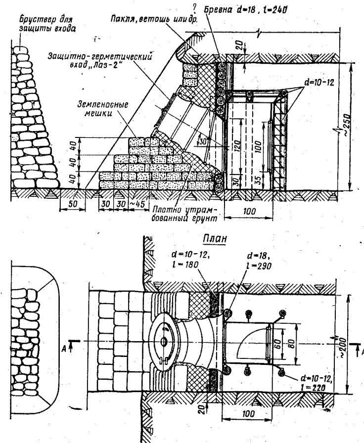
Рис. 219. Оборудование входа в пещеру (выработку) с применением входа «Лаз-2» и БЗМ-57
