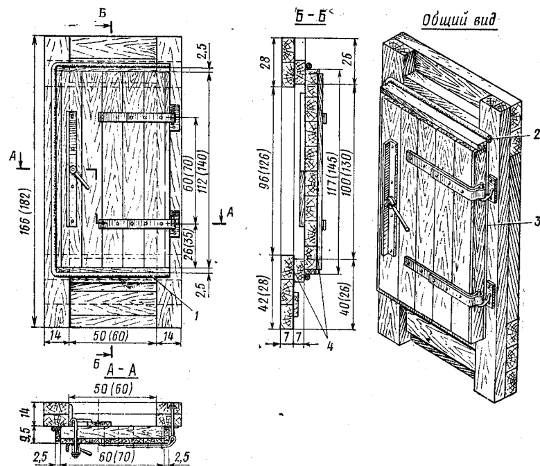
Рис. 244. Блоки дверные БД-50 (БД-60); масса 120 кг (145 кг): 1 — герметизирующий валик из парусины водоупорной пропитки с набивкой ветошью, паклей, отходами капронового волокна; 2 — герметизирующий валик d=40 мм; 3 — герметизирующий валик d=20 мм; 4 — рулонный материал в два слоя
