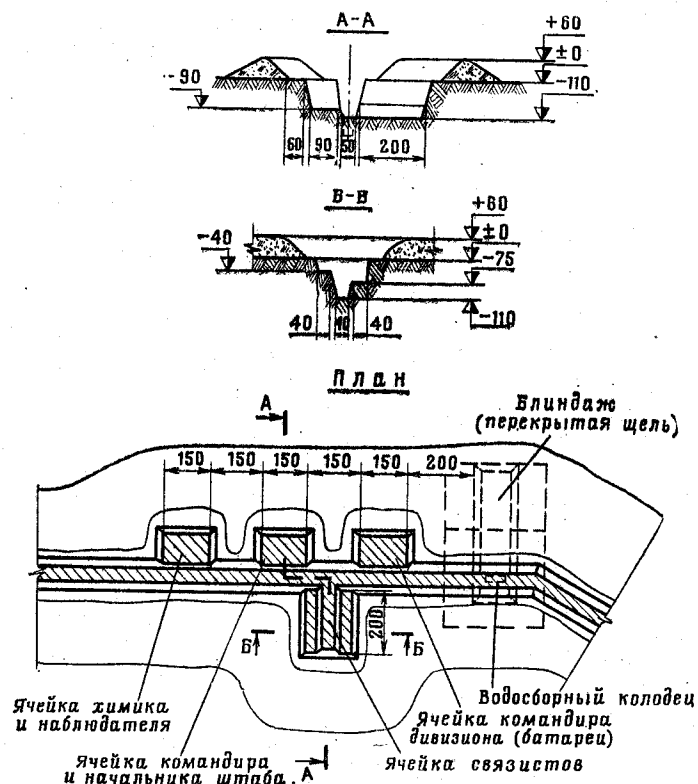
Рис. 92. Открытое сооружение для наблюдения командира батальона Объем вынутого грунта 14 м³. На устройство сооружения без блиндажа требуется 16 чел.-час.
