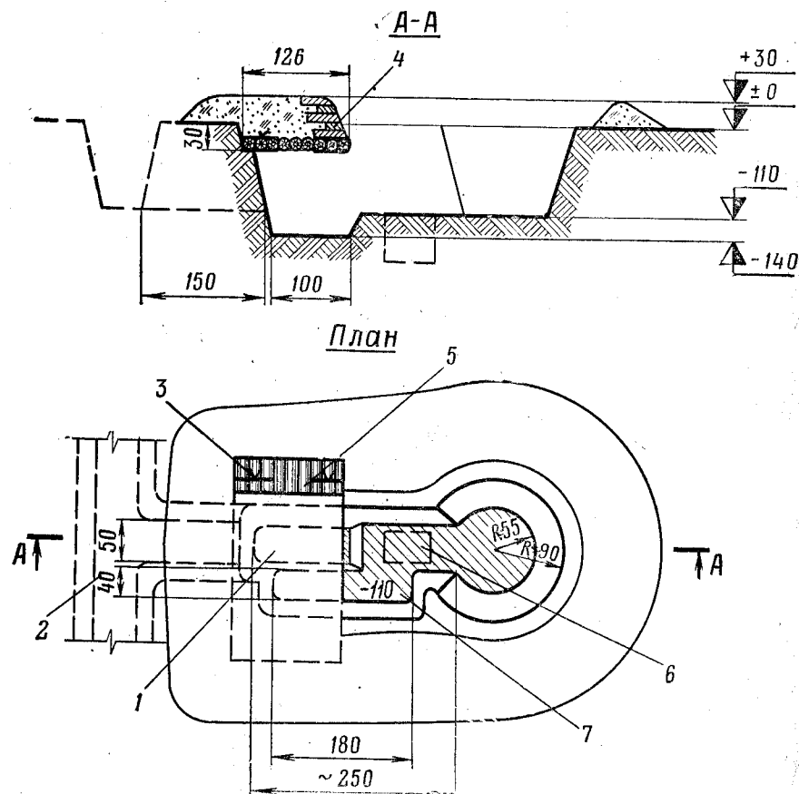
Рис. 385. Окоп для стрелка-зенитчика с нишей на одного человека:
