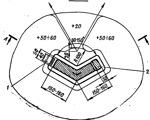
Рис. 8. Окоп для стрельбы из пулемета стоя
