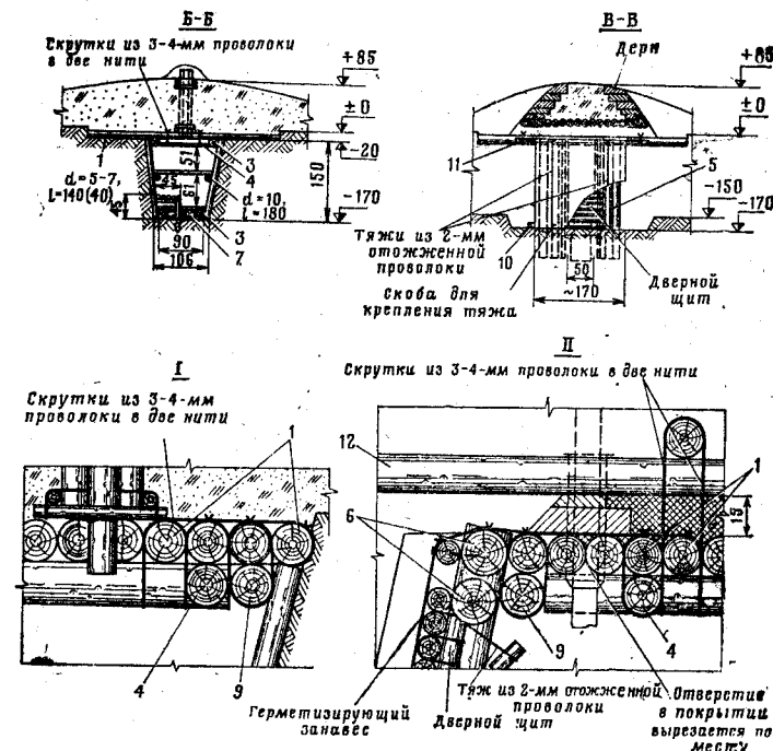
Рис. 116. Блиндаж безрубочной конструкции из лесоматериала на отделение (экипаж)
