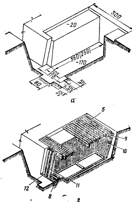
Рис. 314. Последовательность сборки блиндажа безврубочной конструкции из лесоматериала на отделение (экипаж):
