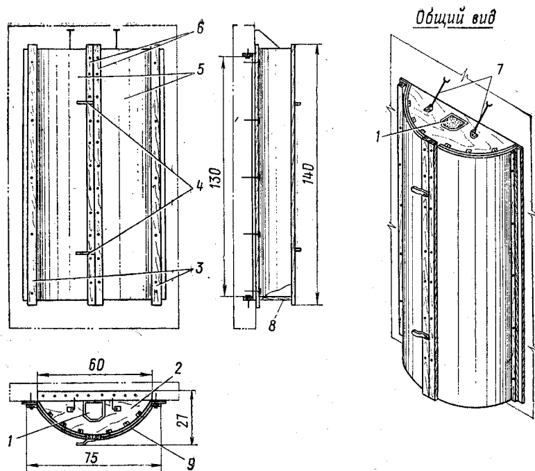
Рис. 248. Раздвижная герметическая дверь РГД; масса 10,2 кг: 1 — клапан; 2 — верхний сегмент; 3 — боковые планки; 4 — запоры; 5 — полотнища; 6 — средние планки; 7 — крючки; 8 — нижний сегмент; 9 — направляющее ребро
