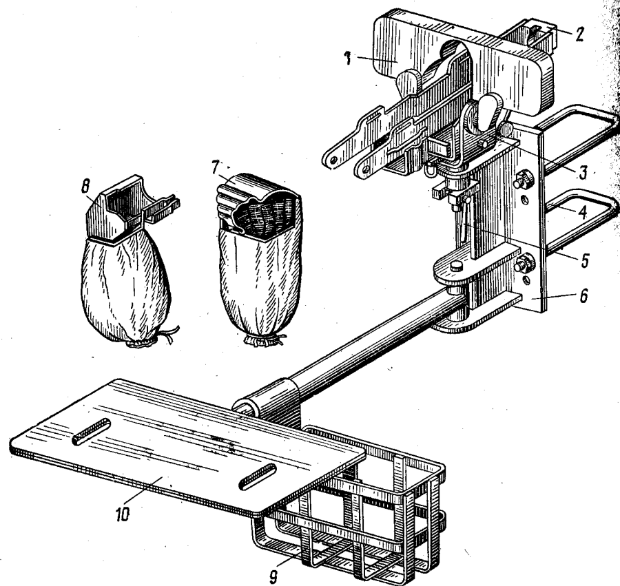
Рис. 254. Настенный пулеметный станок НПС; масса 46 кг: 1 — щиток; 2 — вкладыш; 3 — вертлюг; 4 — скоба с гайками и шайбами; 5 — рукоятка стопора; 6 — кронштейн; 7 — гильзоуловитель для пулемета РПК и автомата АК; 8 — гильзоуловитель для пулемета ПК; 9 — корзинка; 10 — подлокотник
