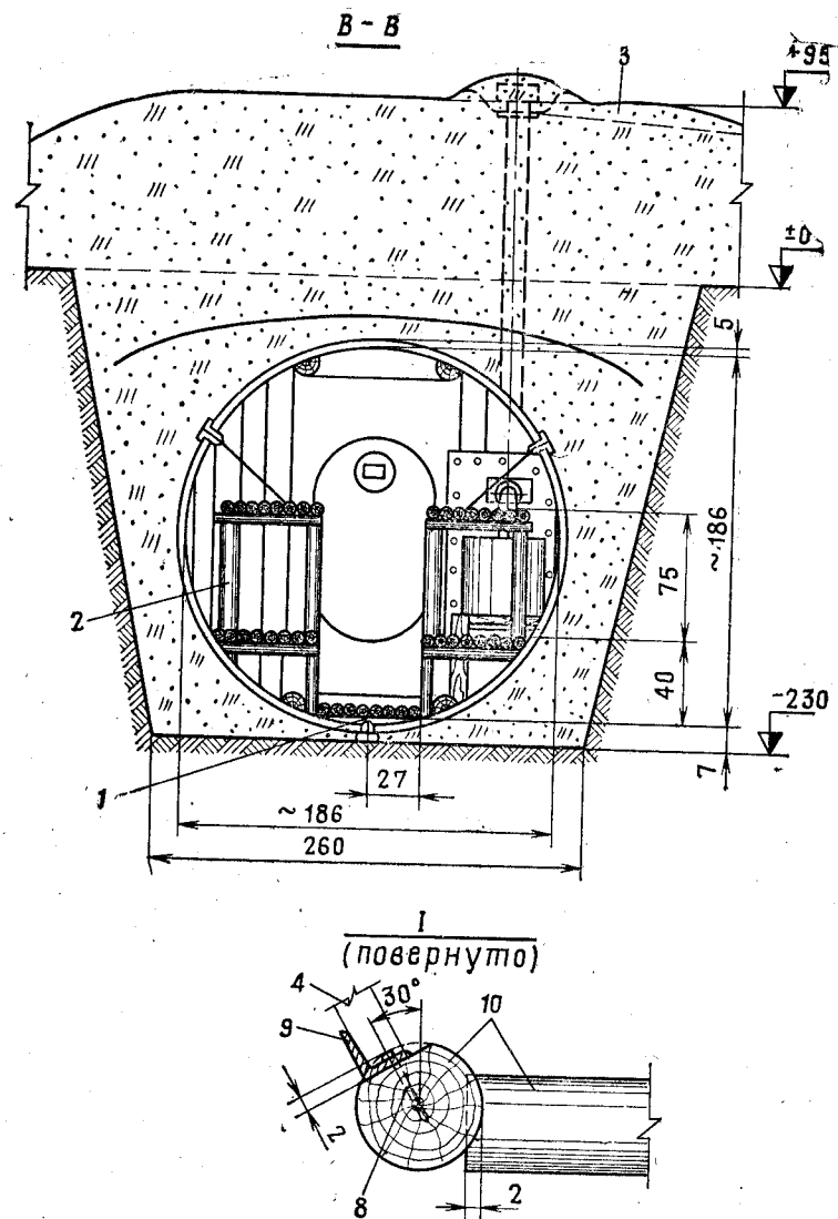
Рис. 395. Убежище из элементов волнистой стали ФВС с входом «Лаз-2» (разрезы, рама Р1, узел 1):
