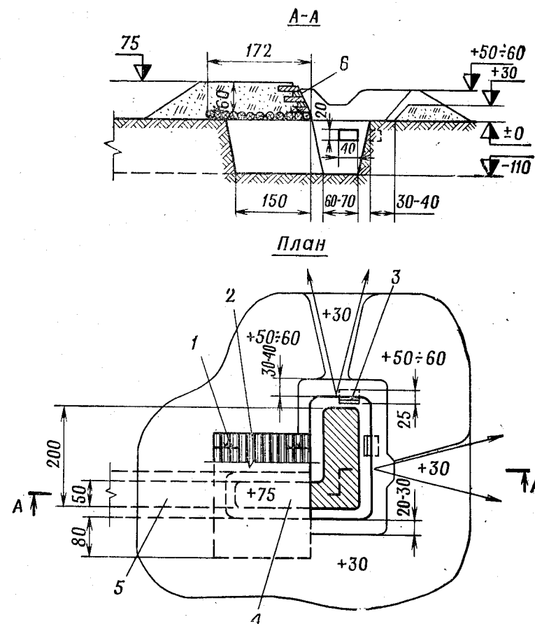
Рис. 386. Окоп для двух стрелков с нишей на два человека: 1 — скрутка из 3—4-мм проволоки в четыре нити; 2 — покрытие d=12-14 см, l=200-300 см; 3 — ниша для боеприпасов; 4 — ниша на два человека; 5 — траншея; 6 — дерн Объем вынутого грунта 3,4 м 3 . На устройство окопа пехотной лопатой требуется 9,5 чел.-час., саперной лопатой — 7 чел.-час., круглого леса — 0,5 м 3 , проволоки — 1,5 кг Примечание. Покрытие l=300 см принимается в случае возможного использования этих элементов для устройства щели на отделении
