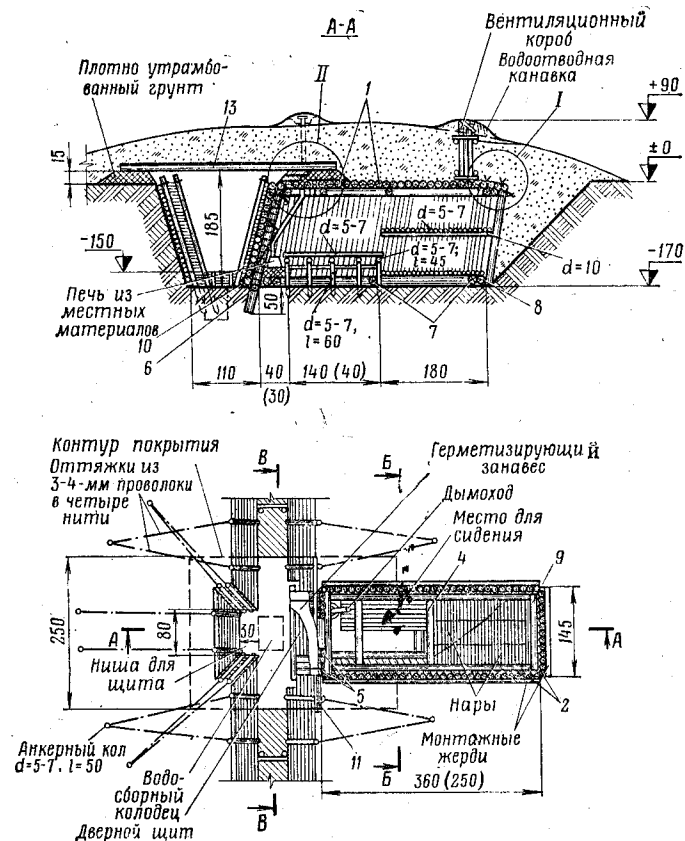
Рис. 207. Блиндаж безврубочной конструкции из лесоматериала в неустойчивых грунтах (план). Объем вынутого грунта 23(17) м³. На устройство блиндажа тр
