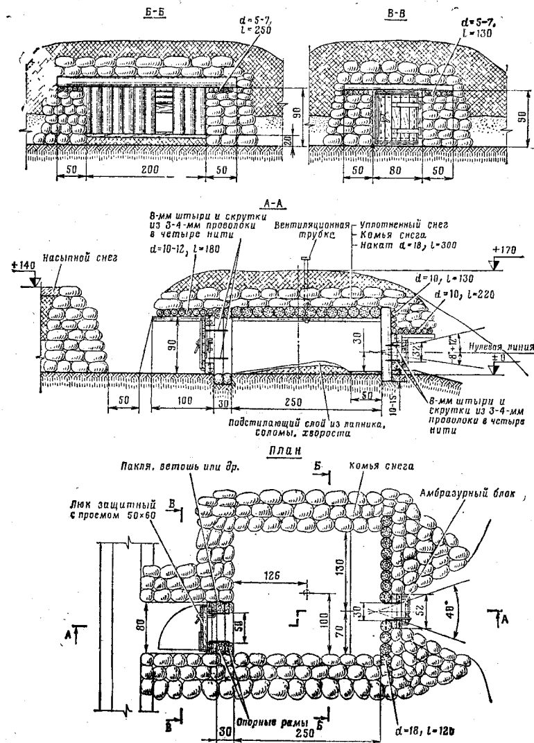
Рис. 194. Сооружение закрытого типа для стрельбы из пулемета лежа. На устройство сооружения требуется 60 чел.-час., снежных комьев — 16,5 \text{ м}^3 , лесоматериала — 2,5 \text{ м}^3 .
