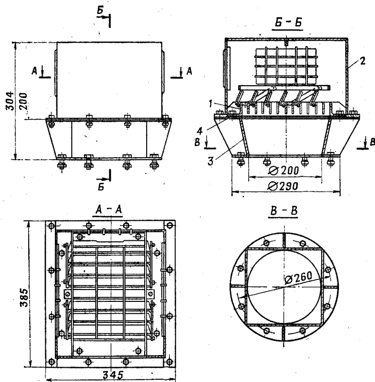
Рис. 280. Вентиляционное защитное устройство МЗС:
