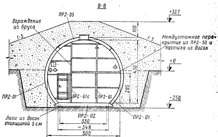
Рис. 139. Сооружение «Панцирь-2ПУ»
