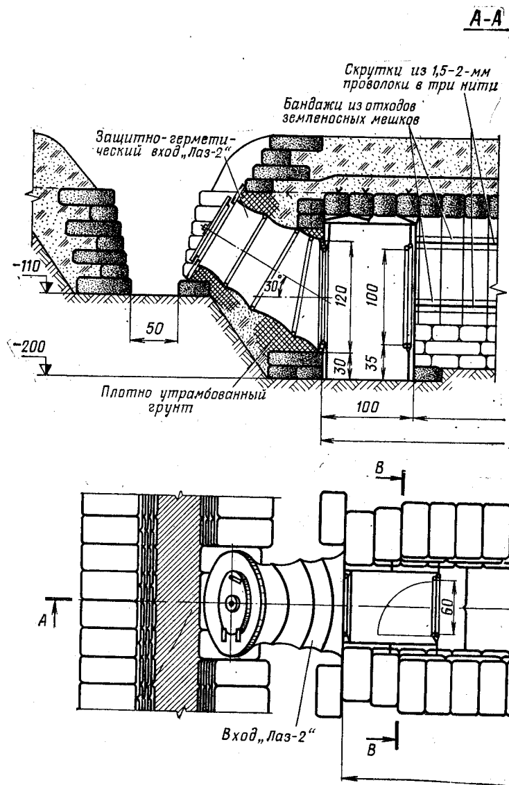
Рис. 233. Убежище из БЗМ-57 и КБМ Объем вынутого грунта 80 м³. На устройство убежища требуется вручную — 175 чел.-час., КБМ — 56 шт., БЗМ-57 — 240 шт.,
