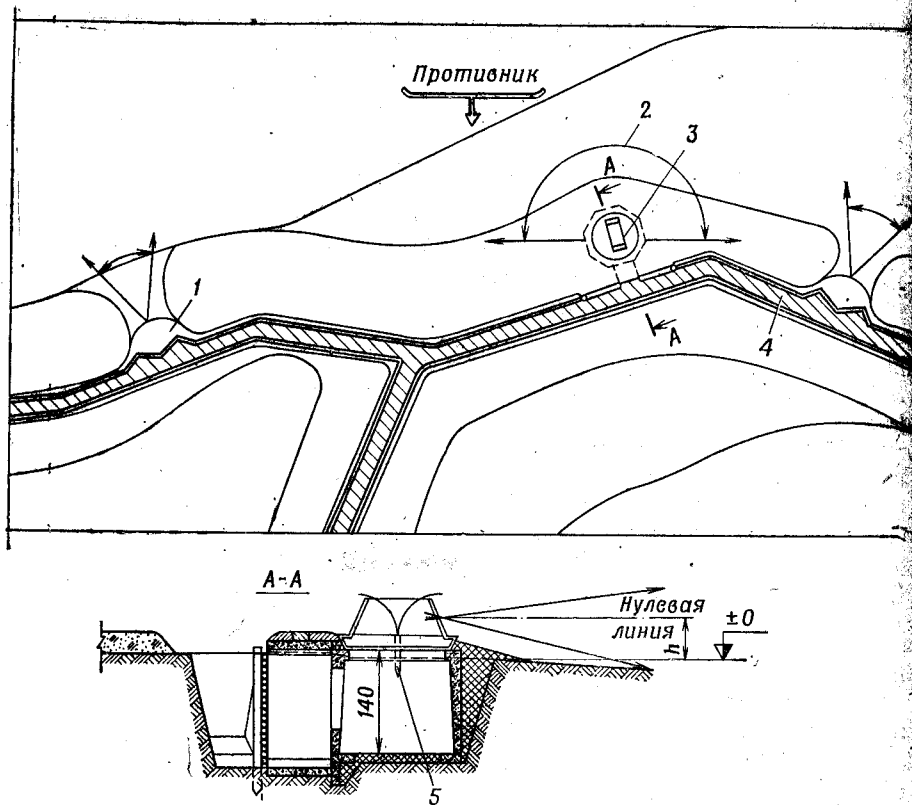
Рис. 303. Посадка пулеметного сооружения СПМ-3 (СПМ-2) на пологом скате или равнинной местности:
