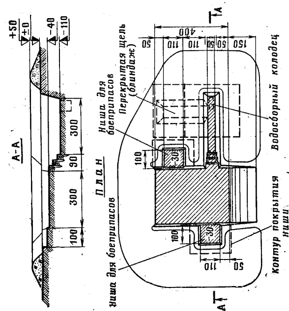
Рис. 80. Окоп для зенитной пулеметной установки ЗПУ-4 Объем вынутого грунта 10 м³. На устройство окопа (без щели) требуется 20 чел.-час., саперной лопатой — 13 чел.-час.
