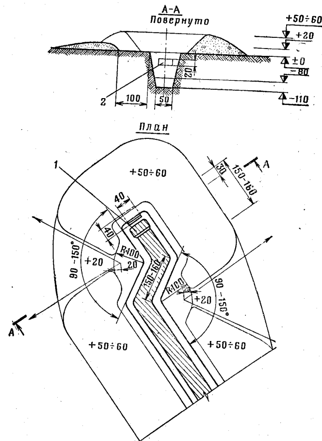
Рис. 20. Вынесенные площадки для стрельбы из пулемета: 1 — ступень для ведения огня в дополнительном секторе; 2 — ниша для боеприпасов
