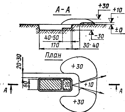
Рис. 2. Окоп для стрельбы из автомата лежа
