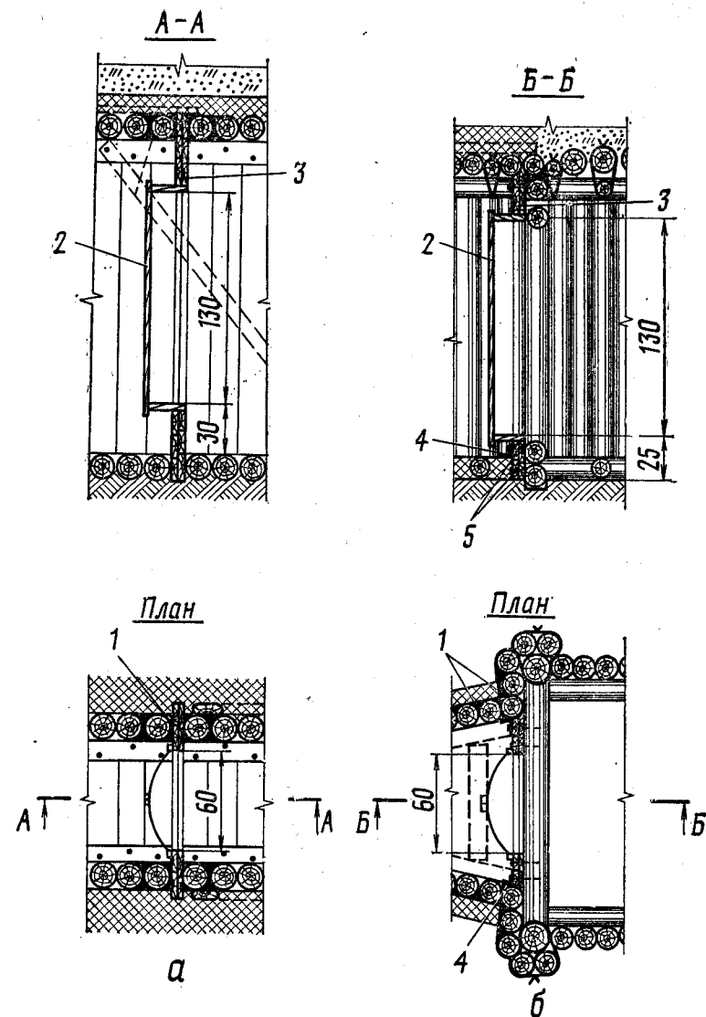
Рис. 253. Установка герметической перегородки во входах сооружений:
