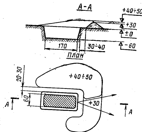
Рис. 3. Окоп для стрельбы из автомата с колена
