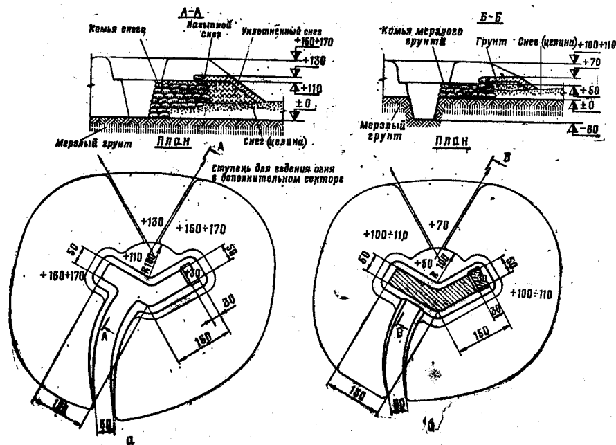
Рис. 190. Окоп для стрельбы из пулемета, устраиваемый в зимних условиях: а — при большом снежном покрове. На устройство окопа требуется 18 чел.-час.; б — при небольшом снежном покрове. Объем вынутого грунта 1,4 м³. На устройство окопа требуется 12 чел.-час.
