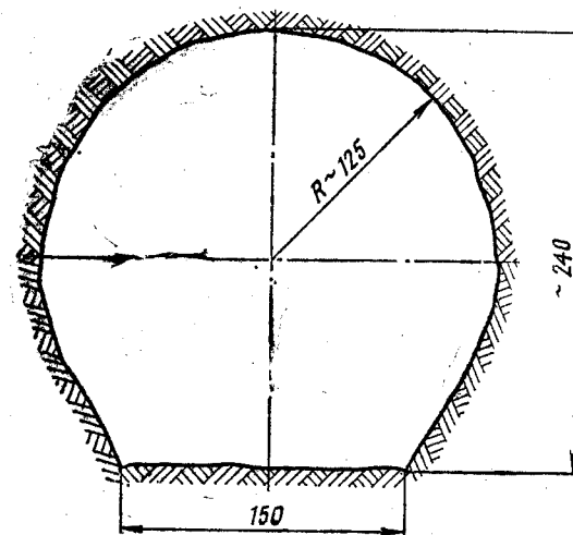
Рис. 330. Поперечное сечение выработки, образуемой проходческим комбайном 2ПУ
