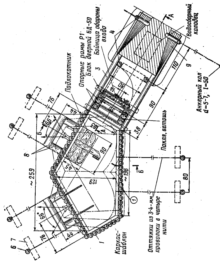
Рис. 31 (лист 1). Пулеметное металлическое сооружение СПМ-1 с основанием из лесоматериала (двухматериальный вариант) Объем вынутого грунта 12 м 3 . На устройство сооружения требуется 48 чел.-час. Металлоизделий — 619 кг, лесоматериала — 2,1 м 3 .
