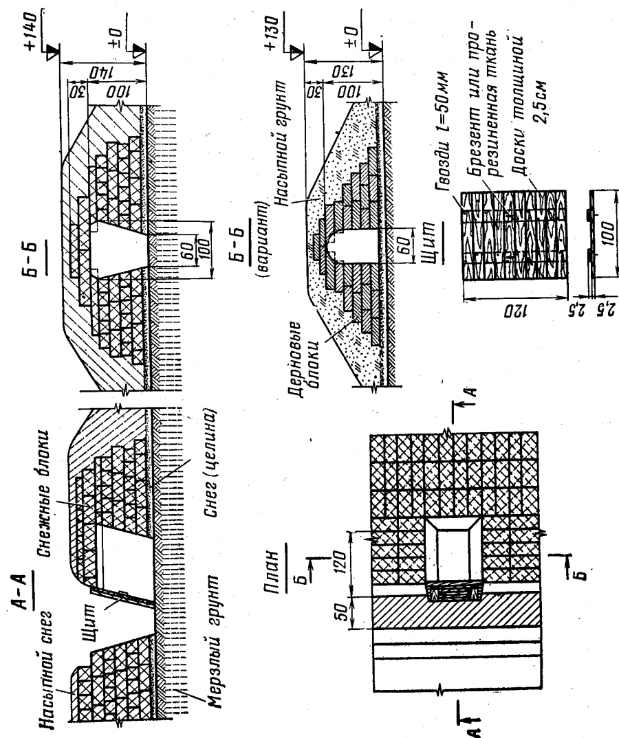
Рис. 197. Ниша для двух человек, устраиваемая из снежных (дерновых) блоков На устройство ниши требуется 60 чел.-час., снежных (дерновых) блоков — 340 шт.
