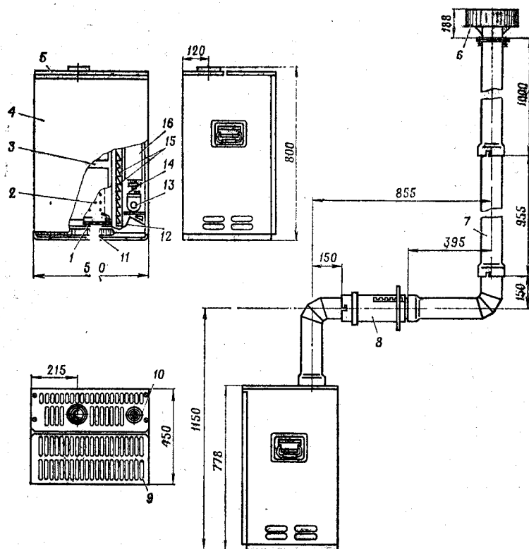
Рис. 282. Многоотопливная отопительная печь МОР-6:
