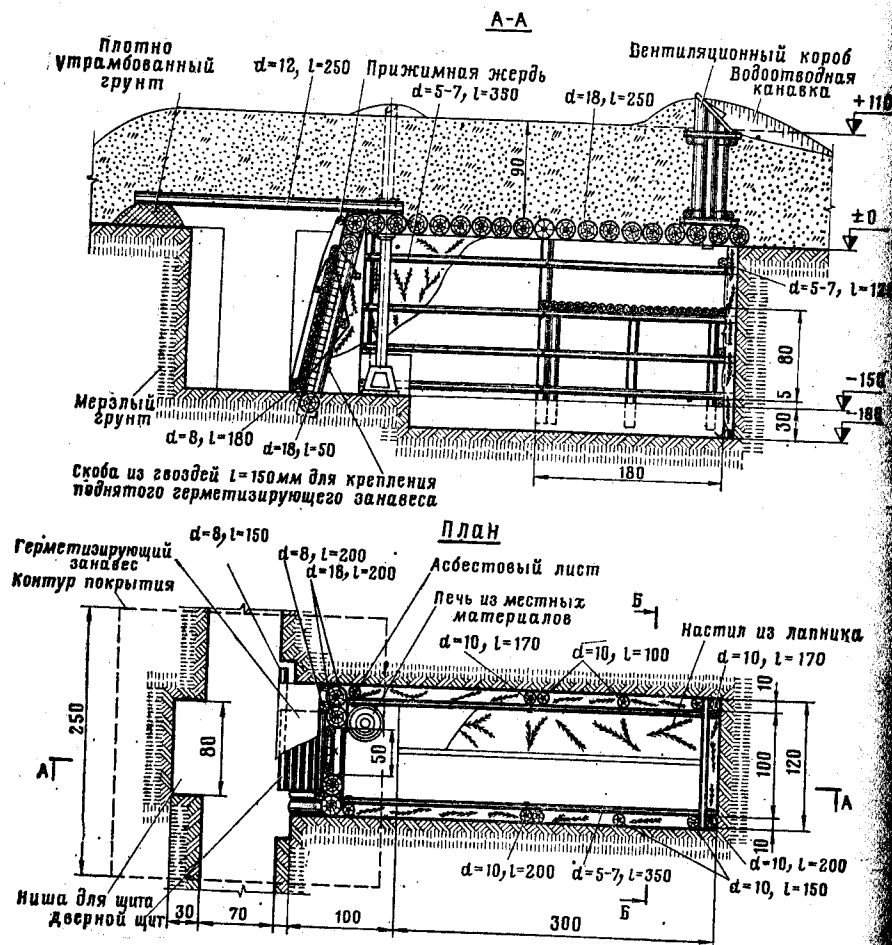
Рис. 200. Блиндаж с перекрытием из круглого леса, возводимый в мерзлом грунте
