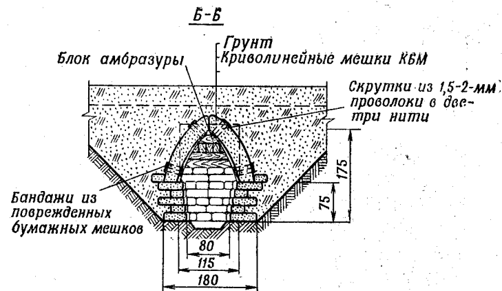
Рис. 223. Сооружение для наблюдения, возводимое из БЗМ-57
