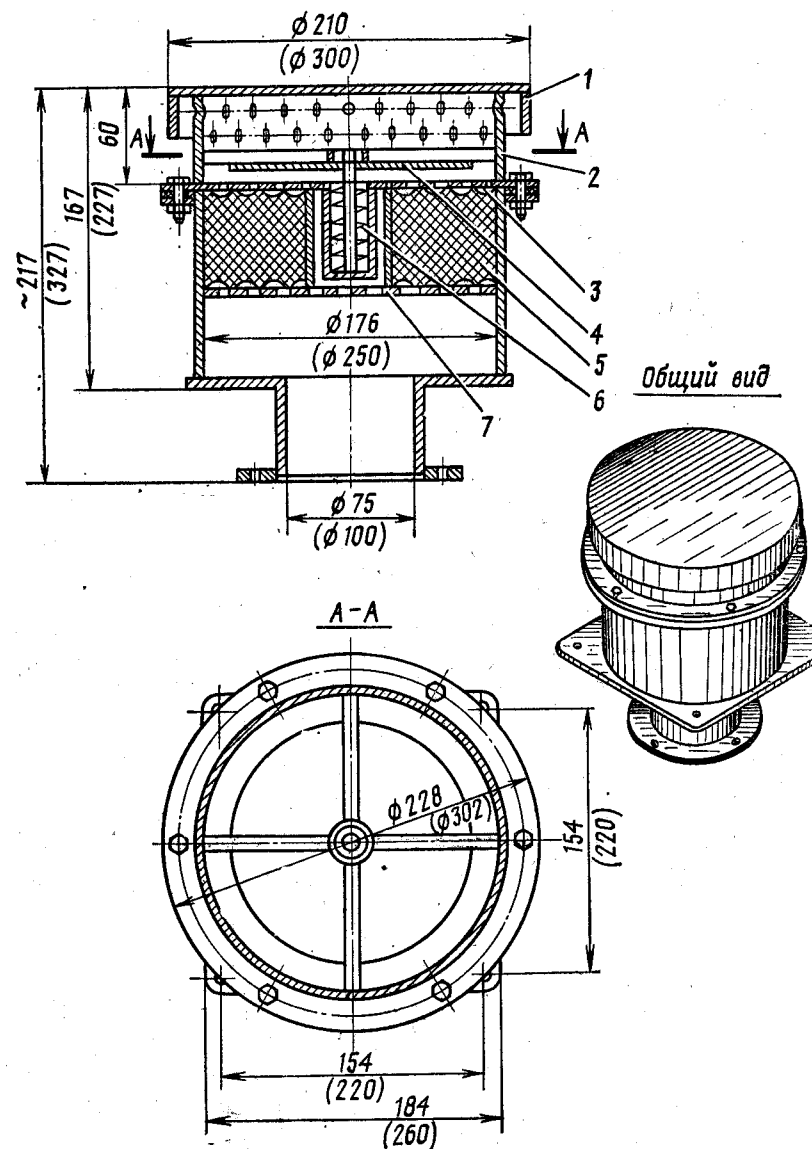
Рис. 279. Вентиляционное защитное устройство ВЗУ-50 (ВЗУ-100): 1 — крышка; 2 — корпус; 3 — решетка; 4 — диск-отсекатель; 5 — алюминиевая стружка; 6 — пружина; 7 — сетка фильтра
