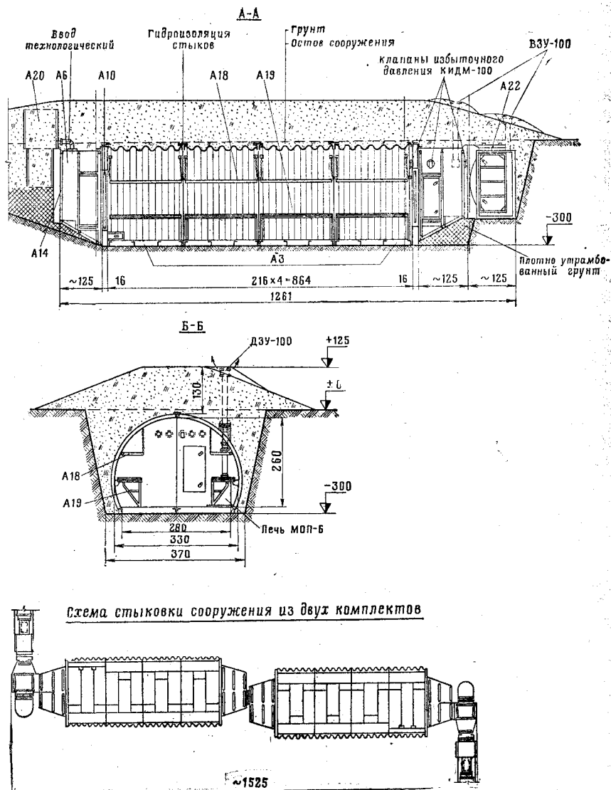
Рис. 137. Сооружение «Бункер» (разрезы, схема стыковки сооружения из двух комплектов)
