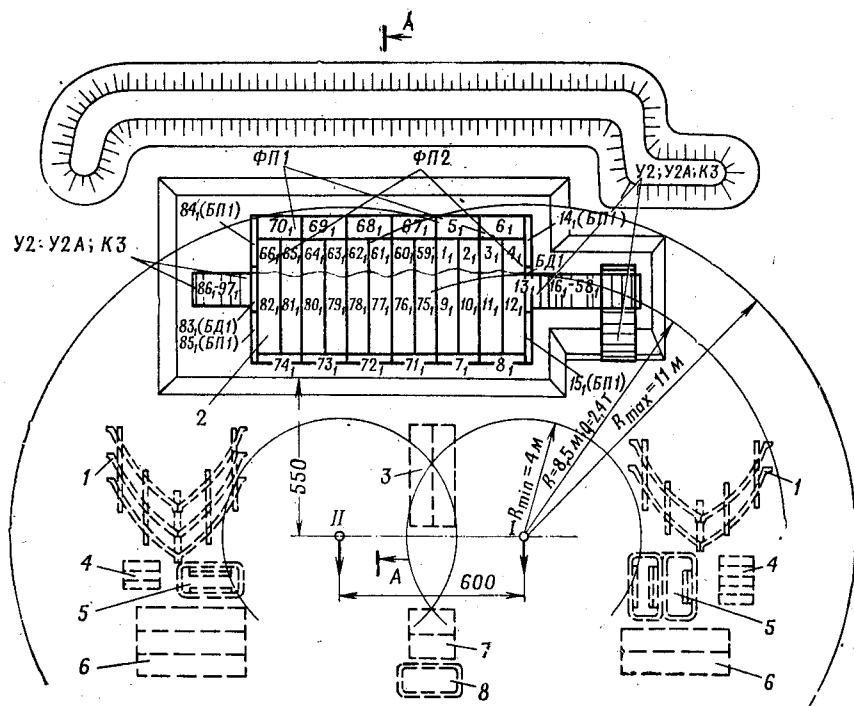
Рис. 324. Последовательность возведения
