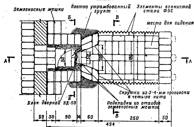
Рис. 231. Блиндаж
