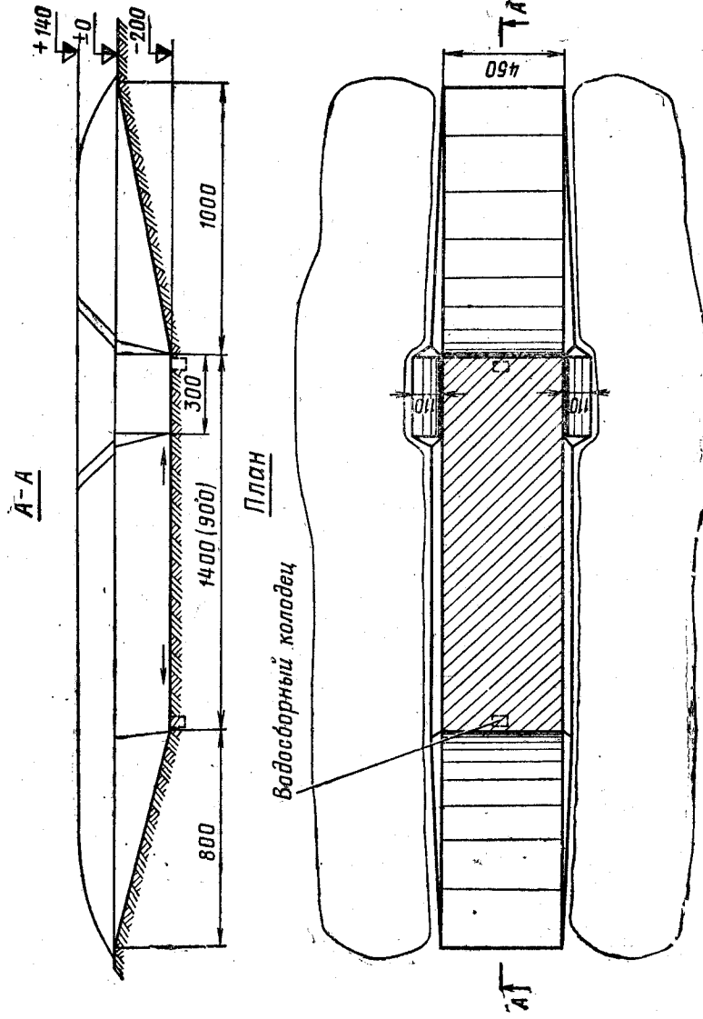
Рис. 48. Окоп для изделий 9П117 (9П117М) и 2П19
