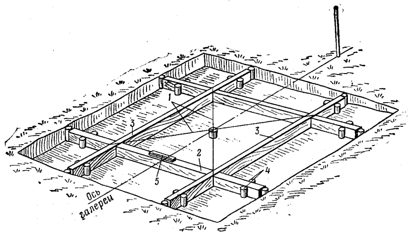
Рис. 329. Установка закладной рамы:
