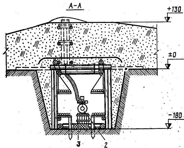
Рис. 269. Монтаж ФВА-50/25 в убежище безврубной конструкции: 1 — ВЗУ-50; 2 — ФВА-50/25; 3 — упаковочный ящик; 4 — плотно утрамбованный грунт
