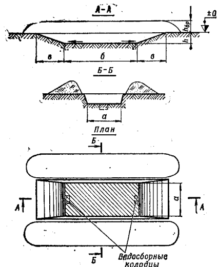
Рис. 127. Укрытия для командно-штабных и специальных машин (на две машины)
